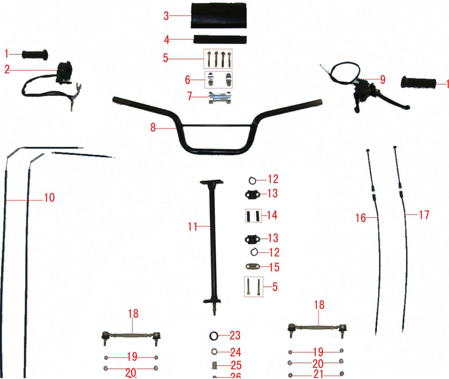
Fig 6: Styringssystem / steering system / Steuerungssystem
