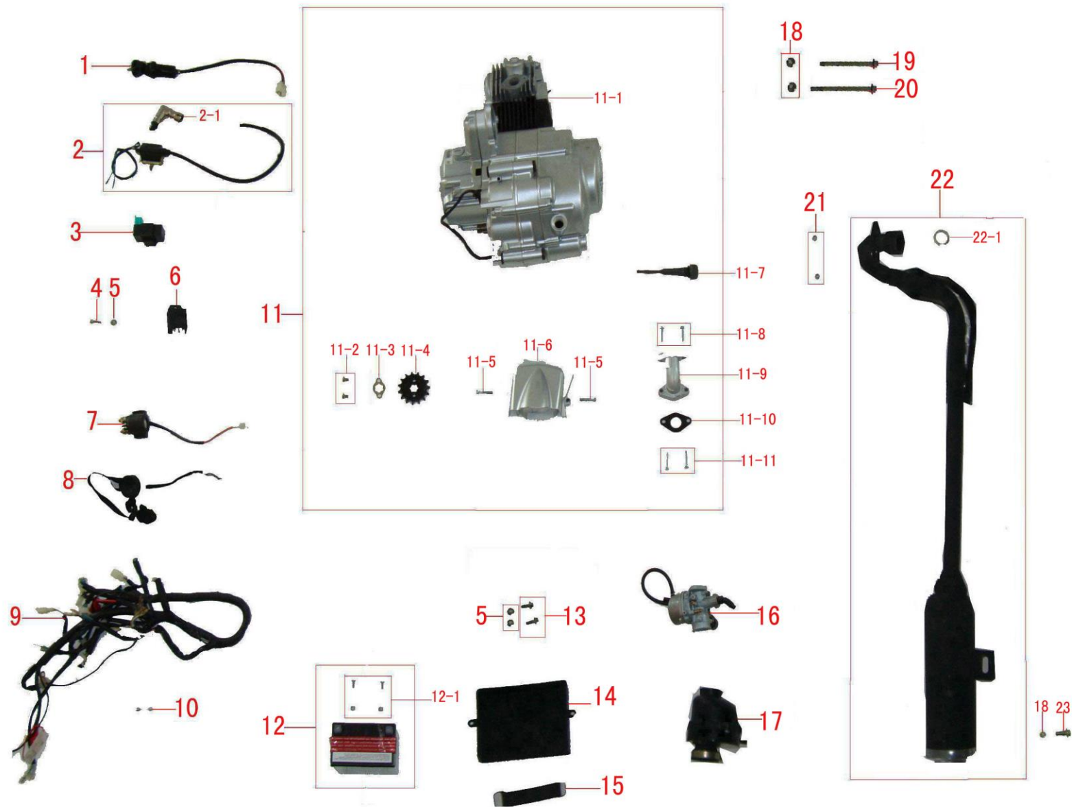
Fig 5: Elektriske dele & motor komponenter / electricals & engine parts / Elektrische Teile & Motorkomponenten
