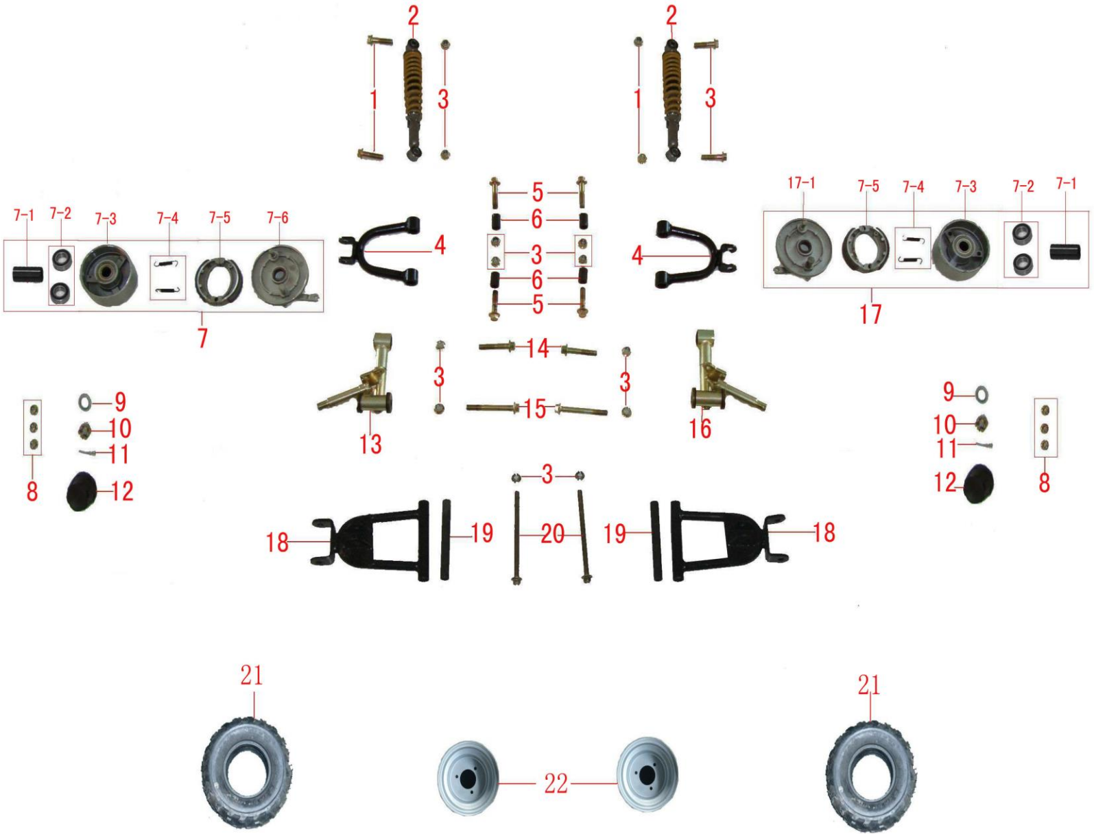
Fig 4: Forhjulsophæng / front suspension / Vorderradaufhängung
