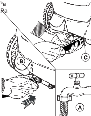
Collegamento idrico.
