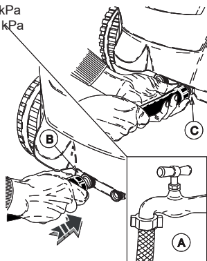
Conexión hídrica.
