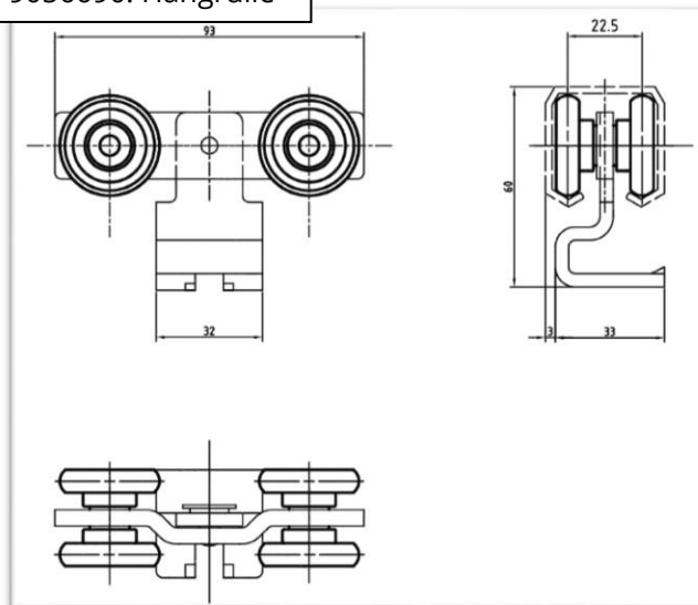
9056690: Hängrulle
