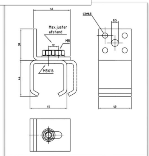
9056694: Mittkonsol
