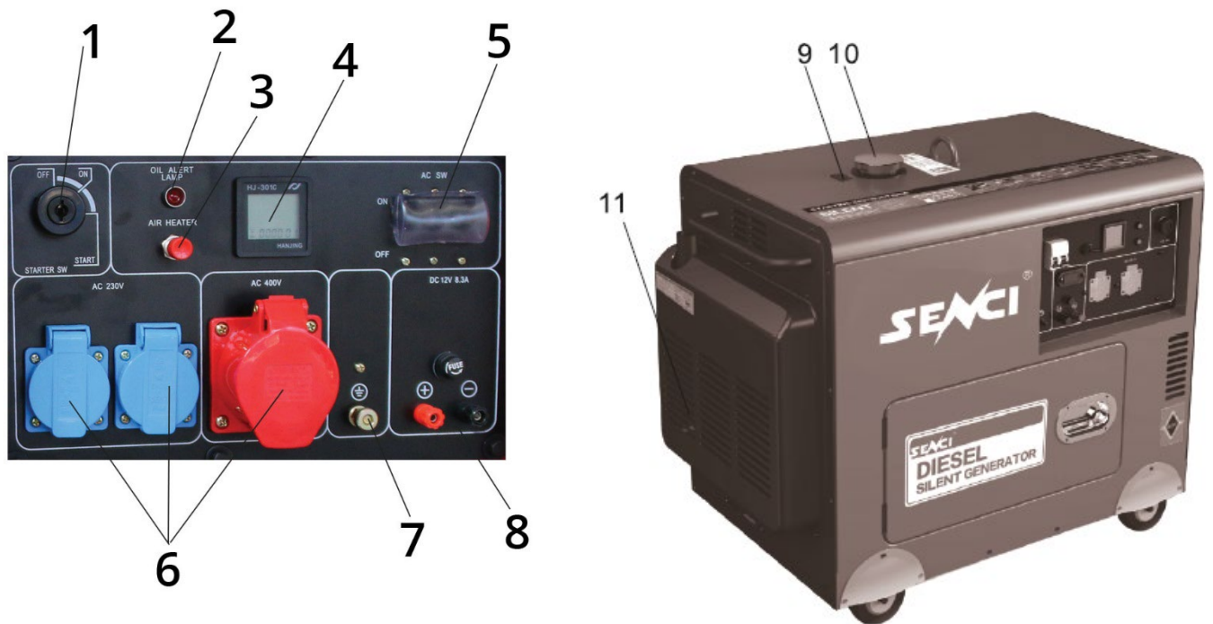
Das oben abgebildete Paneel gehört zum 3-Phasen-Modell mit 2 x 230 V Anschluss (blau) und 1 x 400 V Anschluss (rot).
