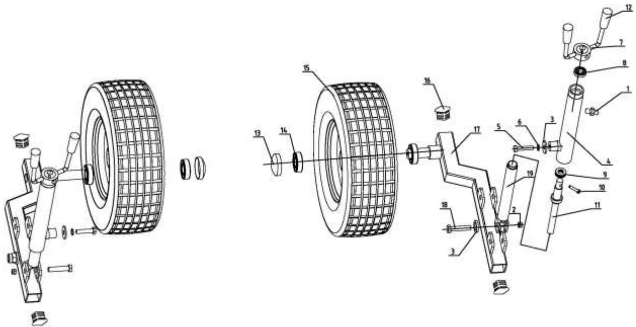
Fig. 3 Hjulupphäng
