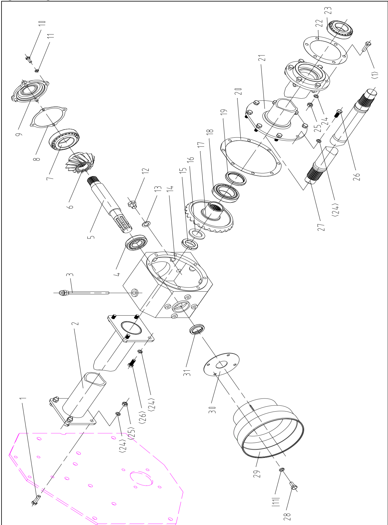
Fig 2 Vinkelgear
