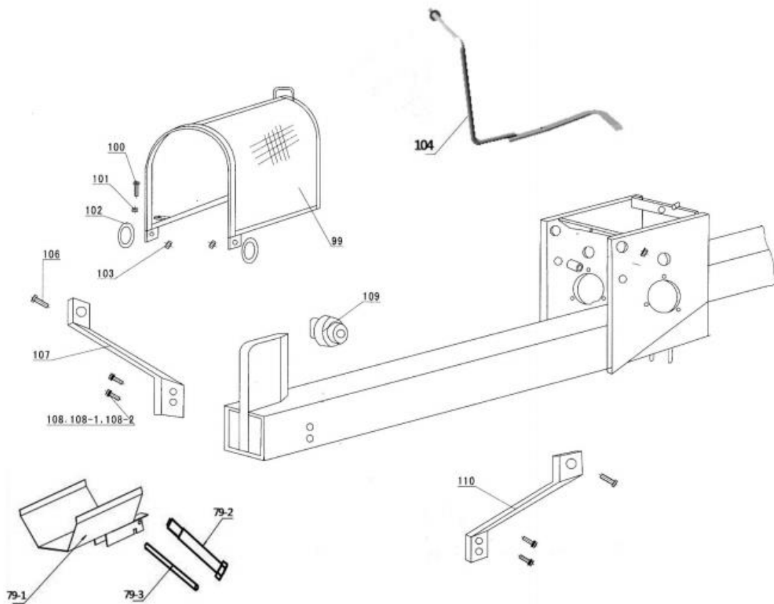
Komponentoversigt, figur 3
