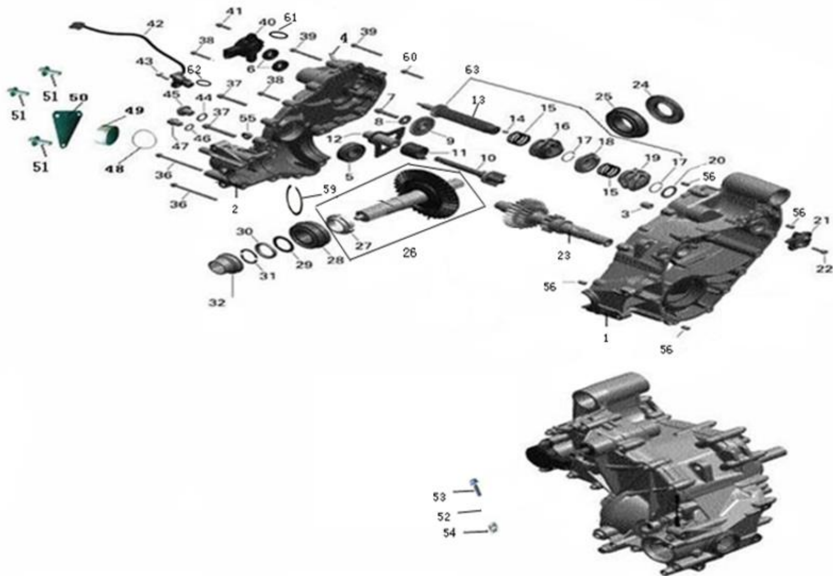
FIGUR 8 – VÄXELLÅDA 1
