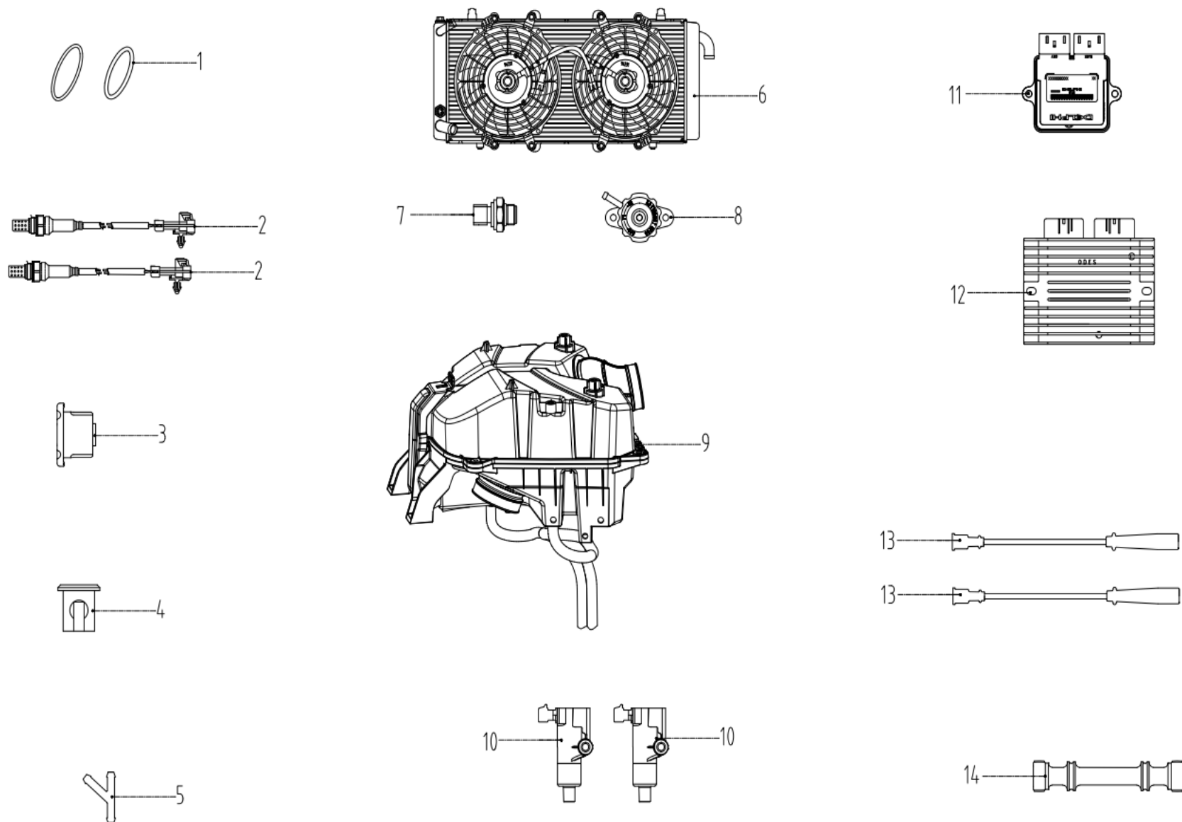
FIGUR 13 – MOTORTILLBEHÖR
