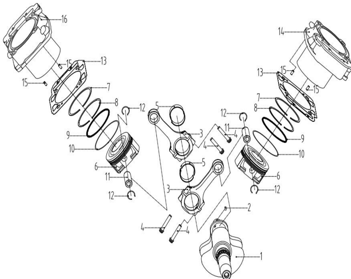
FIGUR 4 – VEVAXEL, KOLV OCH CYLINDER
