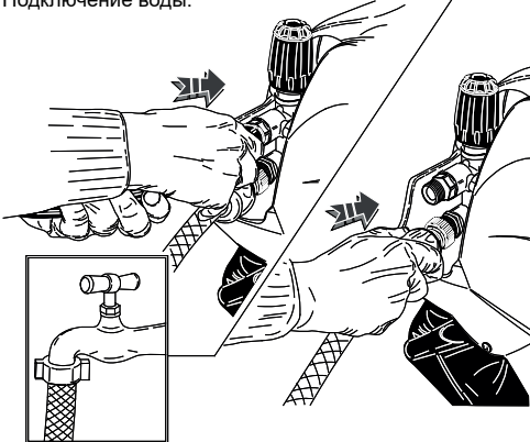
Подключение воды.
