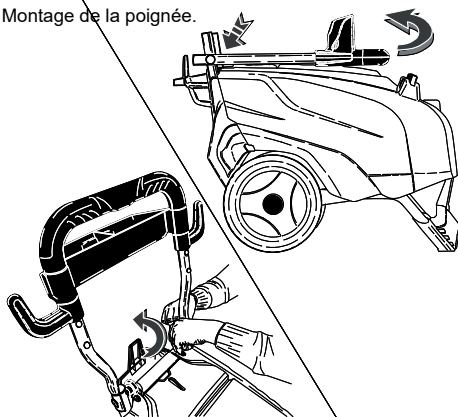
Montage de la poignée.
