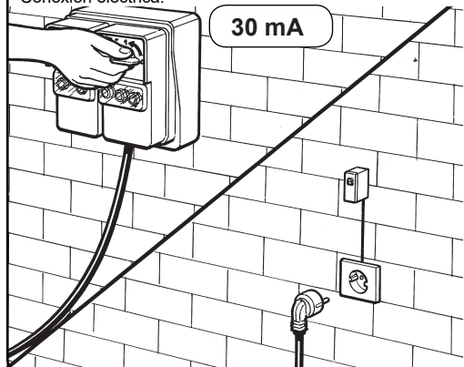
Conexión eléctrica.
