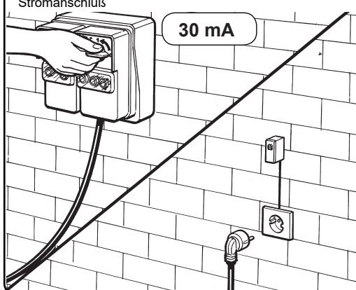
Stromanschluß
