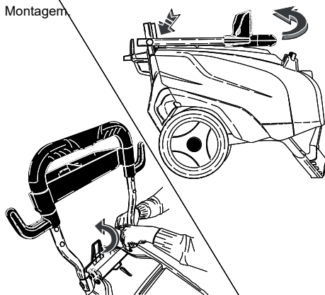
Montagem
