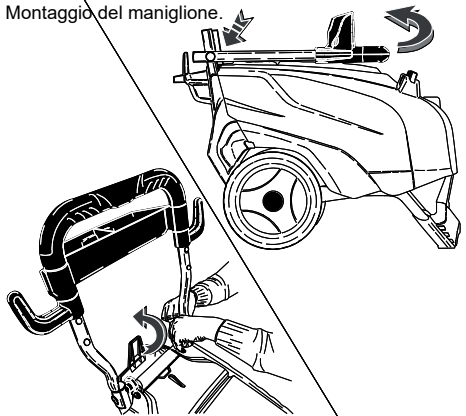
Montaggio del maniglione.
