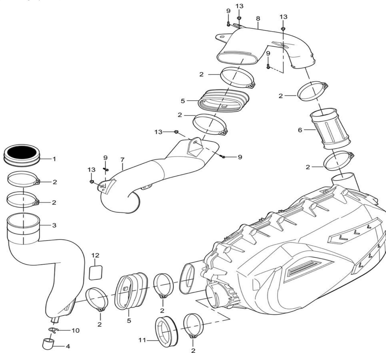
FIGUR 11 – Luftintag CVT (luftintagssystem)
