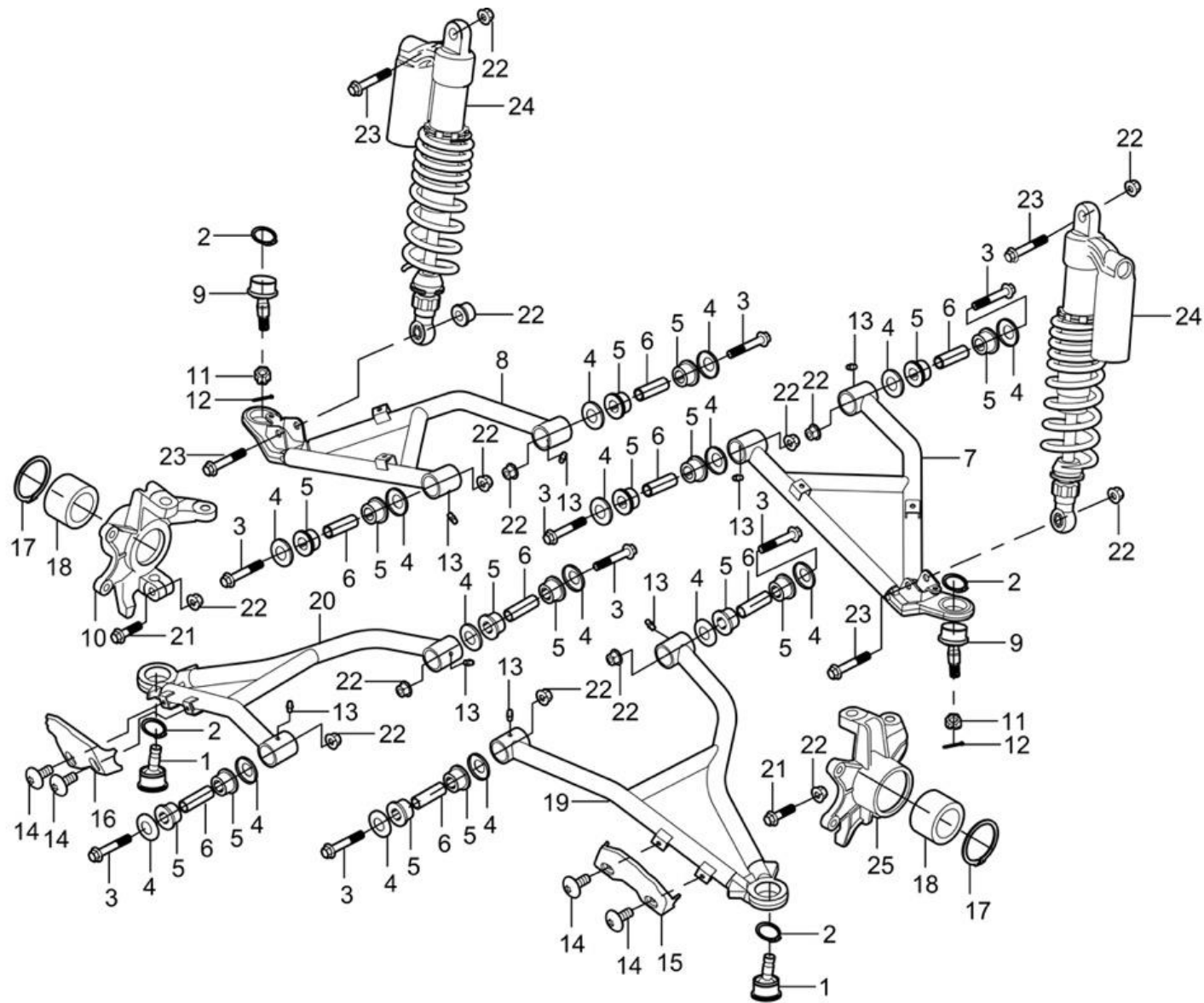
FIGUR 3 – Hjulupphängning, fram (främre fjädringssystem)
