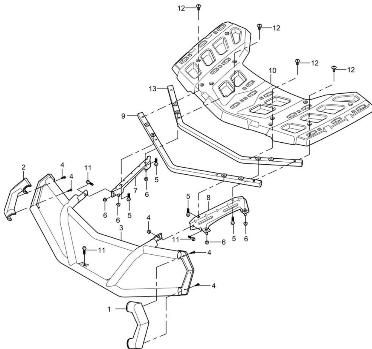
FIGUR 20 – Främre stötfångare, bagagehållare
