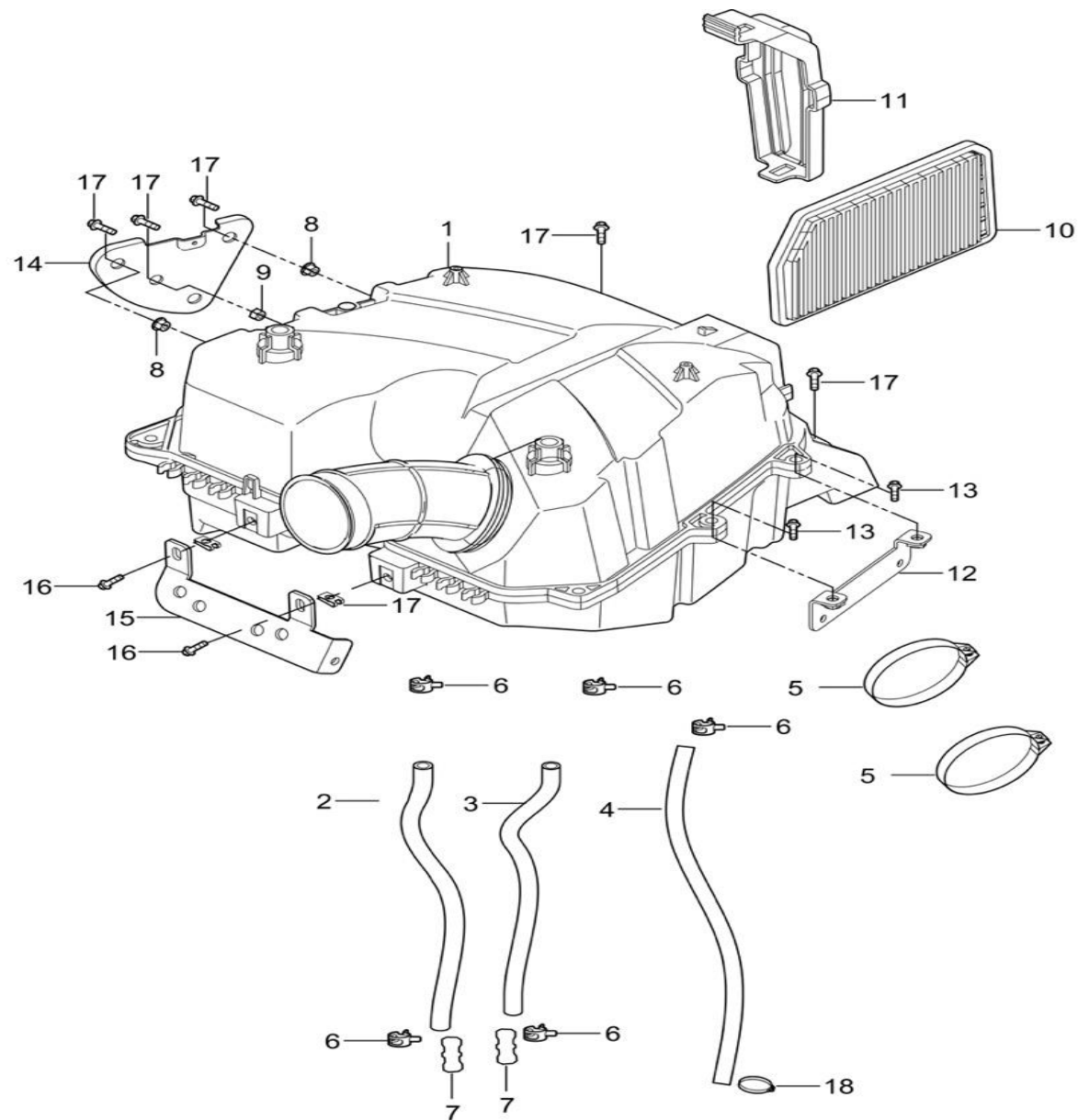
FIGUR 10 – Luftfilter (intagssystem)
