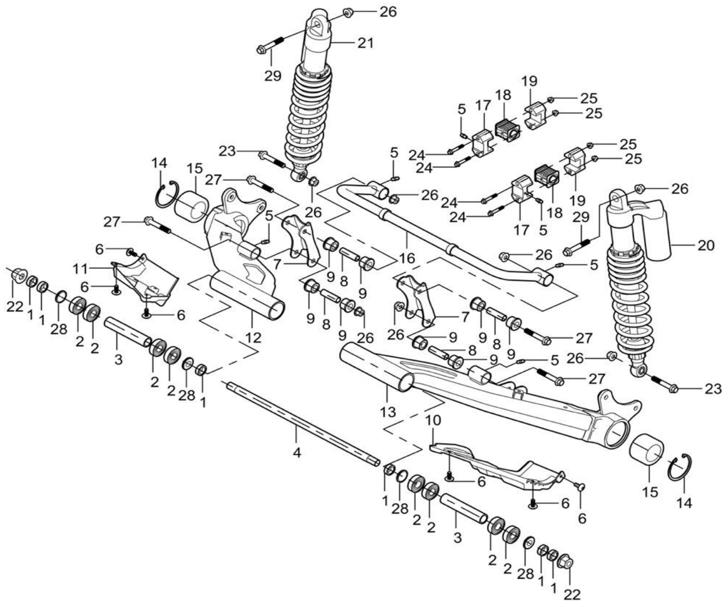
FIGUR 4 – Hjulupphängning, bak (bakfjädringssystem)
