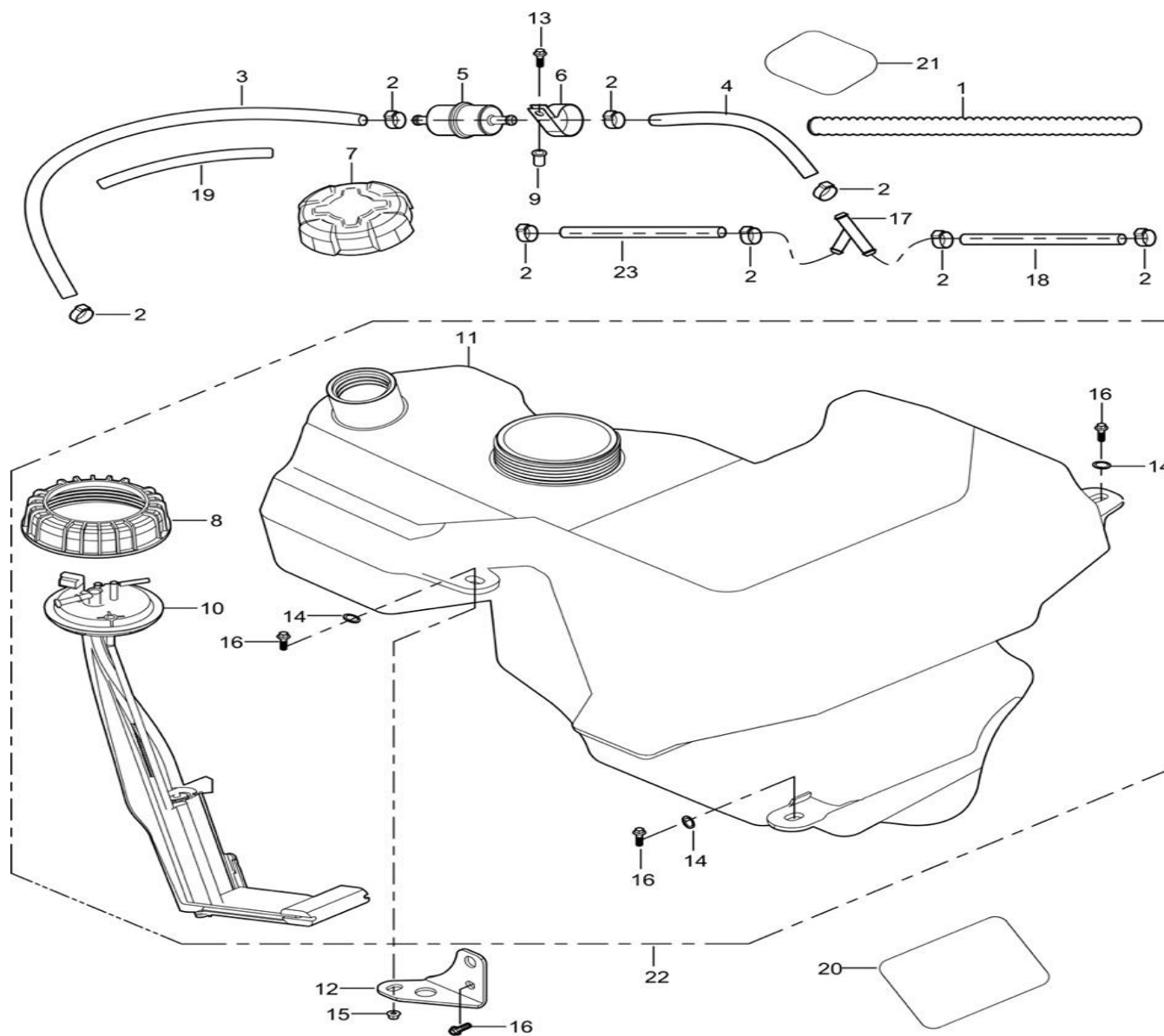
FIGUR 8 – Bränslesystem (bränslesystem)
