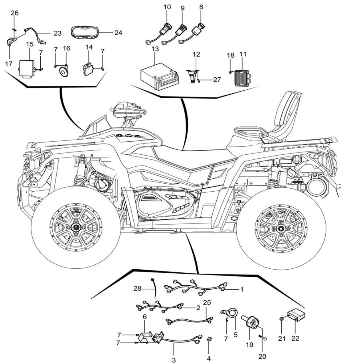
FIGUR 23 – Ledningar, sensorer, kontakter (elektriska delar)
