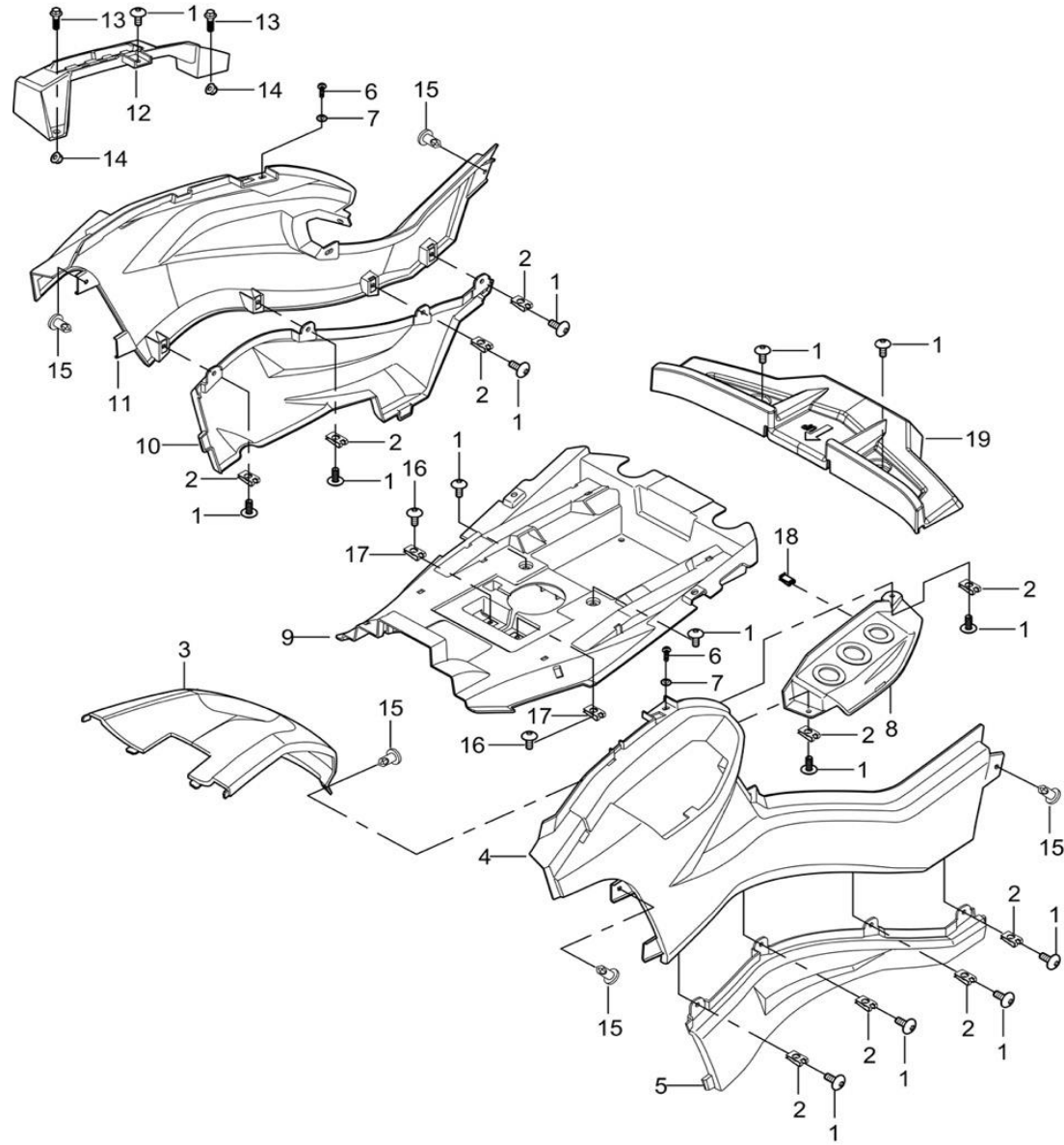
Fig 22: Plastavskärmning sidodelar m.m "kort modell"
