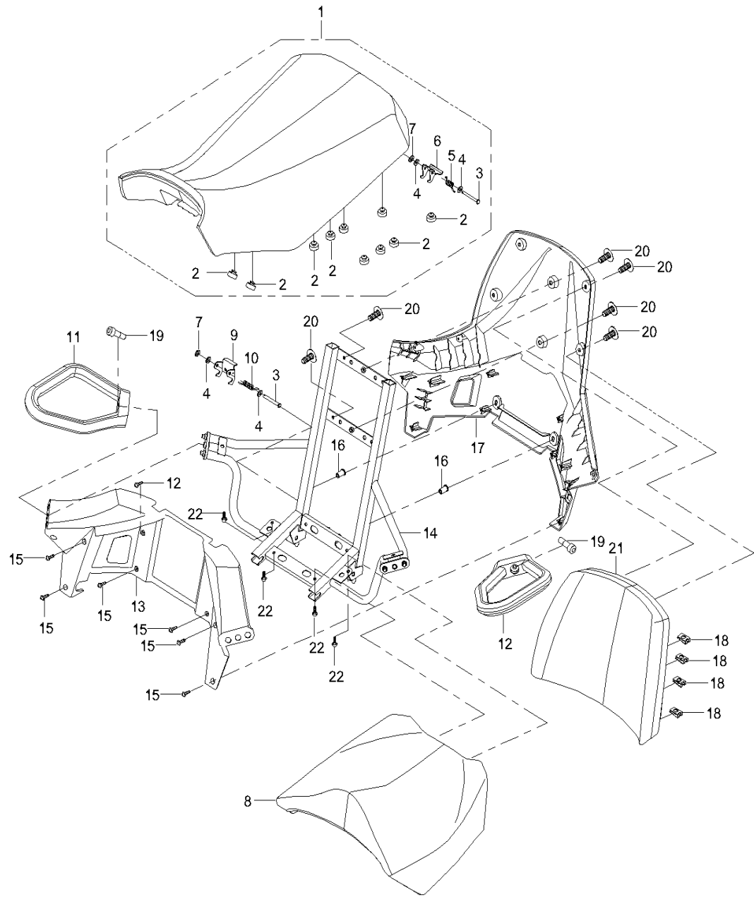
Fig 17: Säte/beslag "lång modell"
