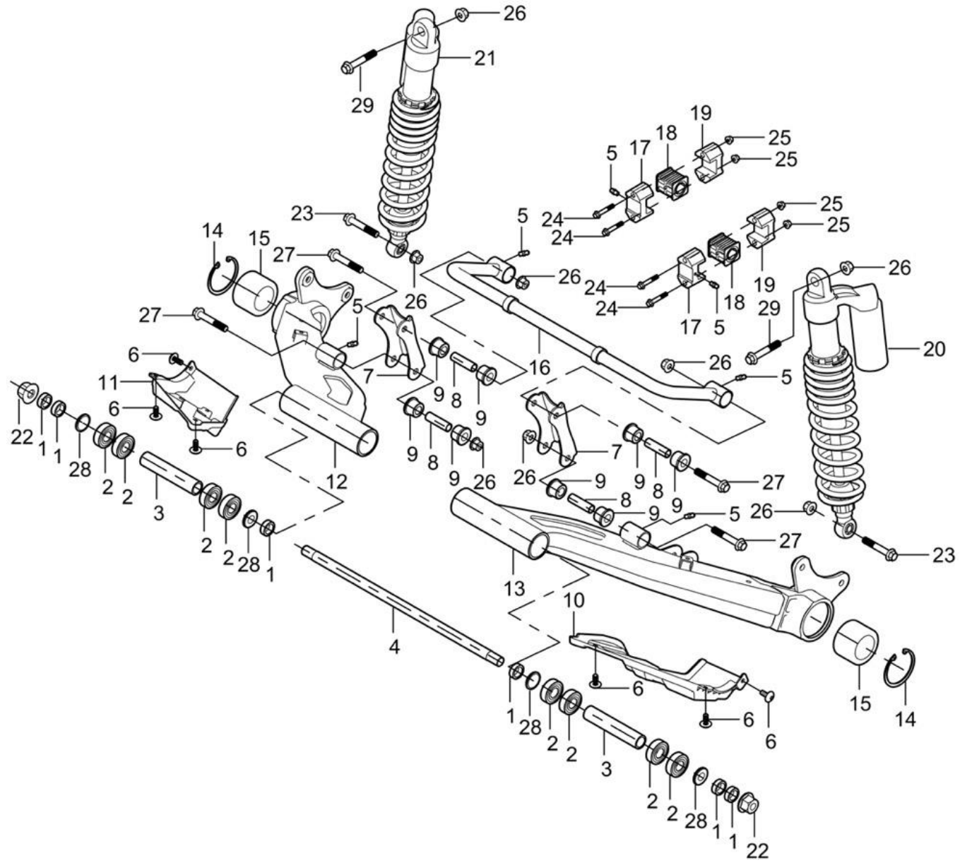
Fig 4: Bakre fjädringssystem
