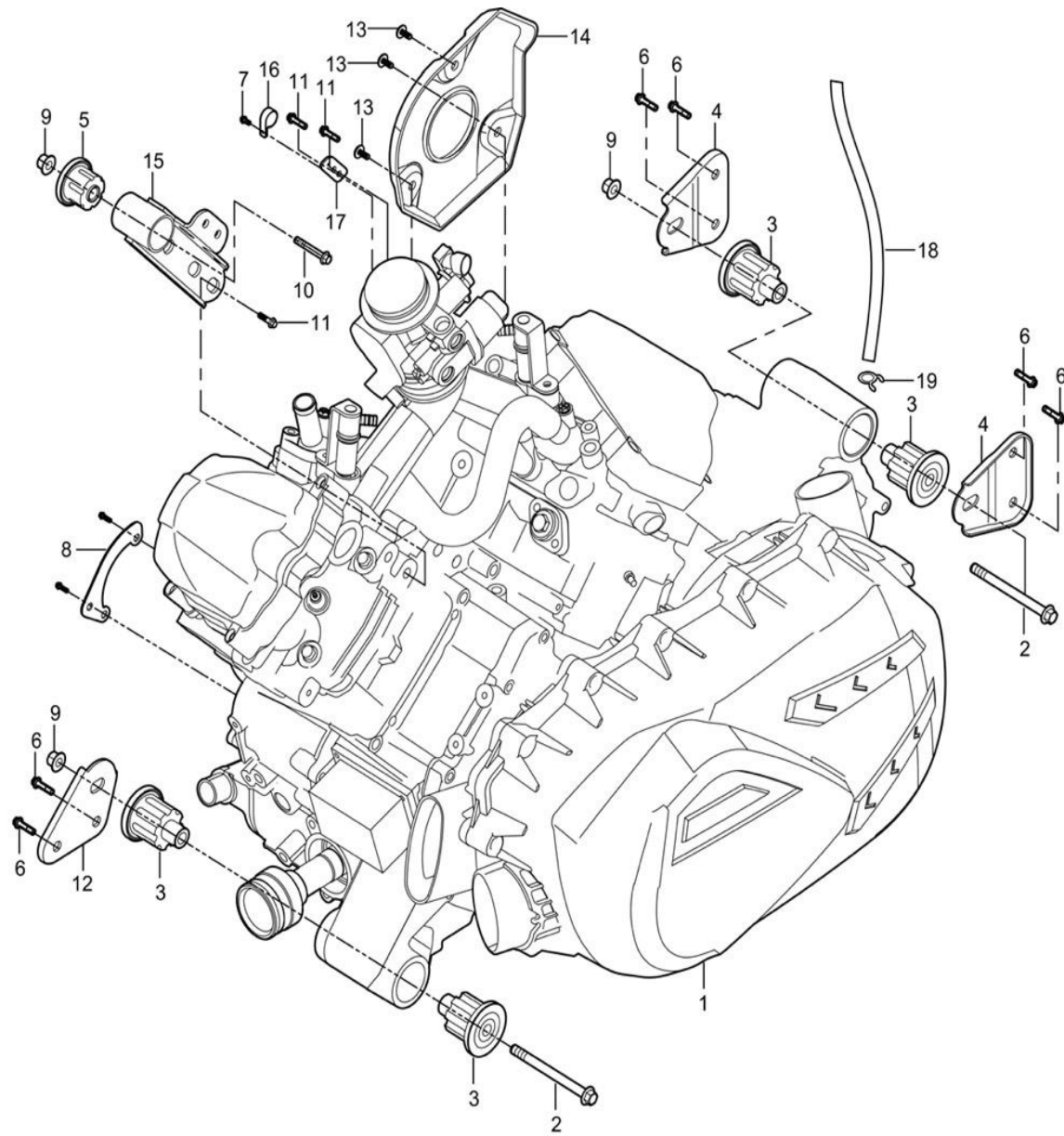
Fig 11: Motor, motorfäste
