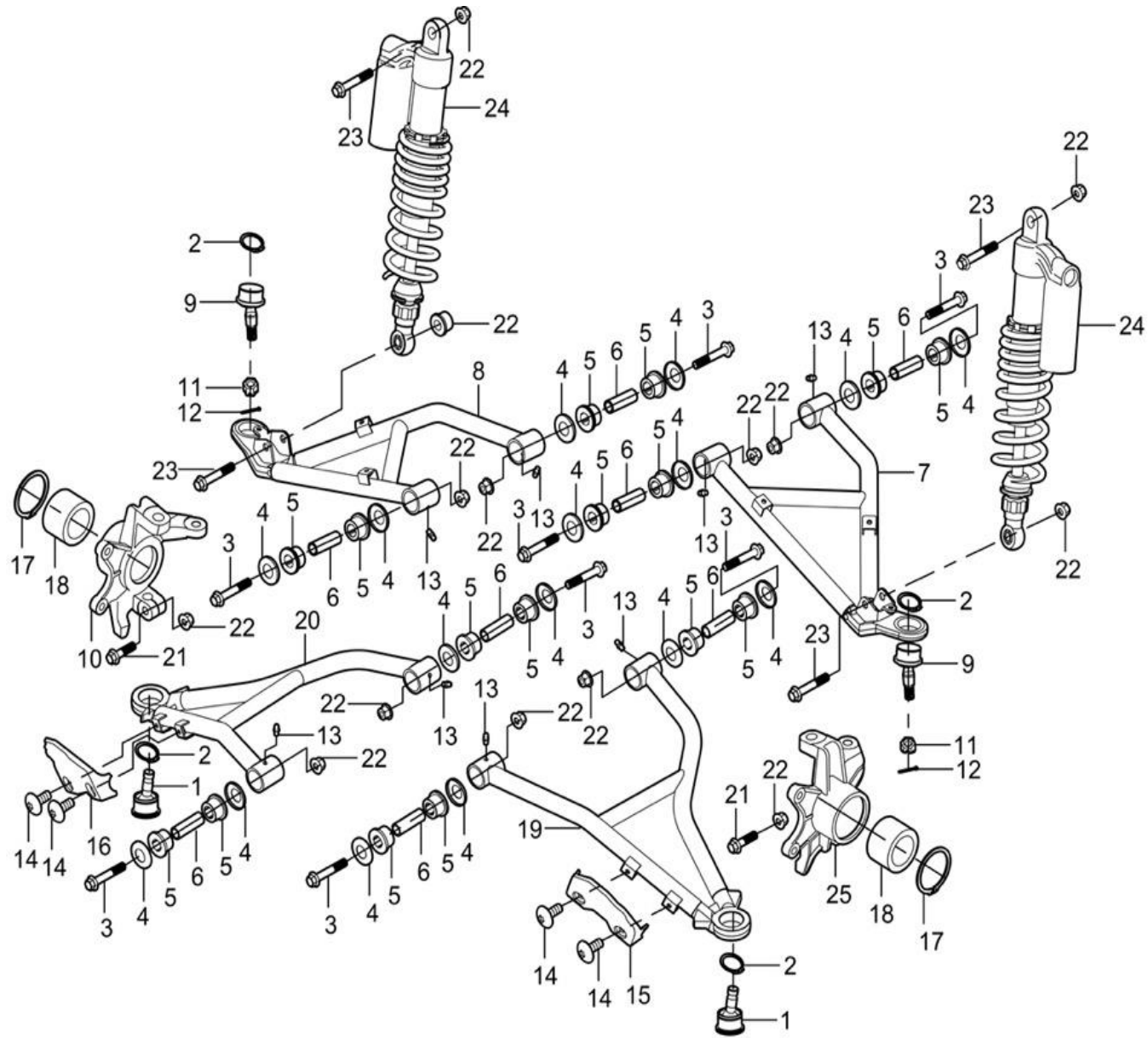
Fig 3: Främre fjädringsystem
