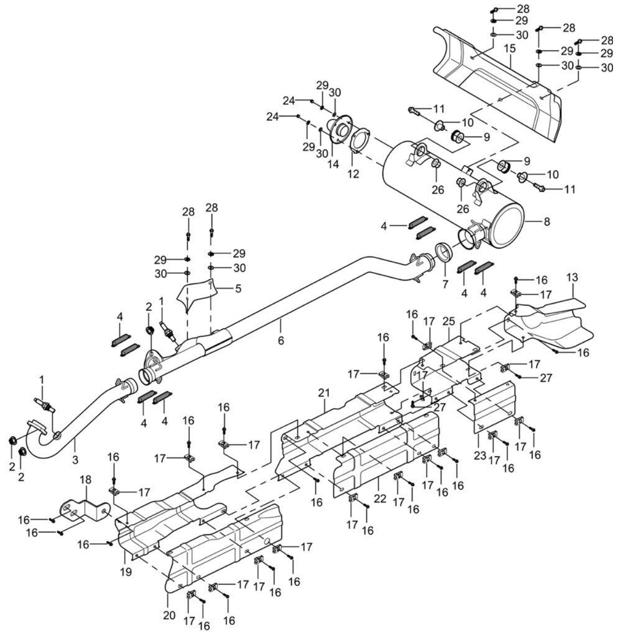
Fig 15: Avgassystemet "lång"
