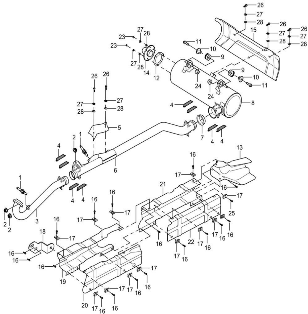
Fig 16: Avgassystemet "kort"
