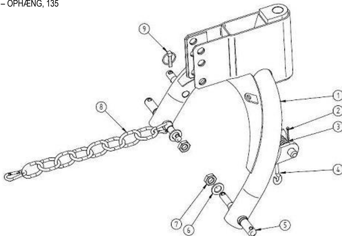
FIGUR 4 – OPHÆNG, 135
