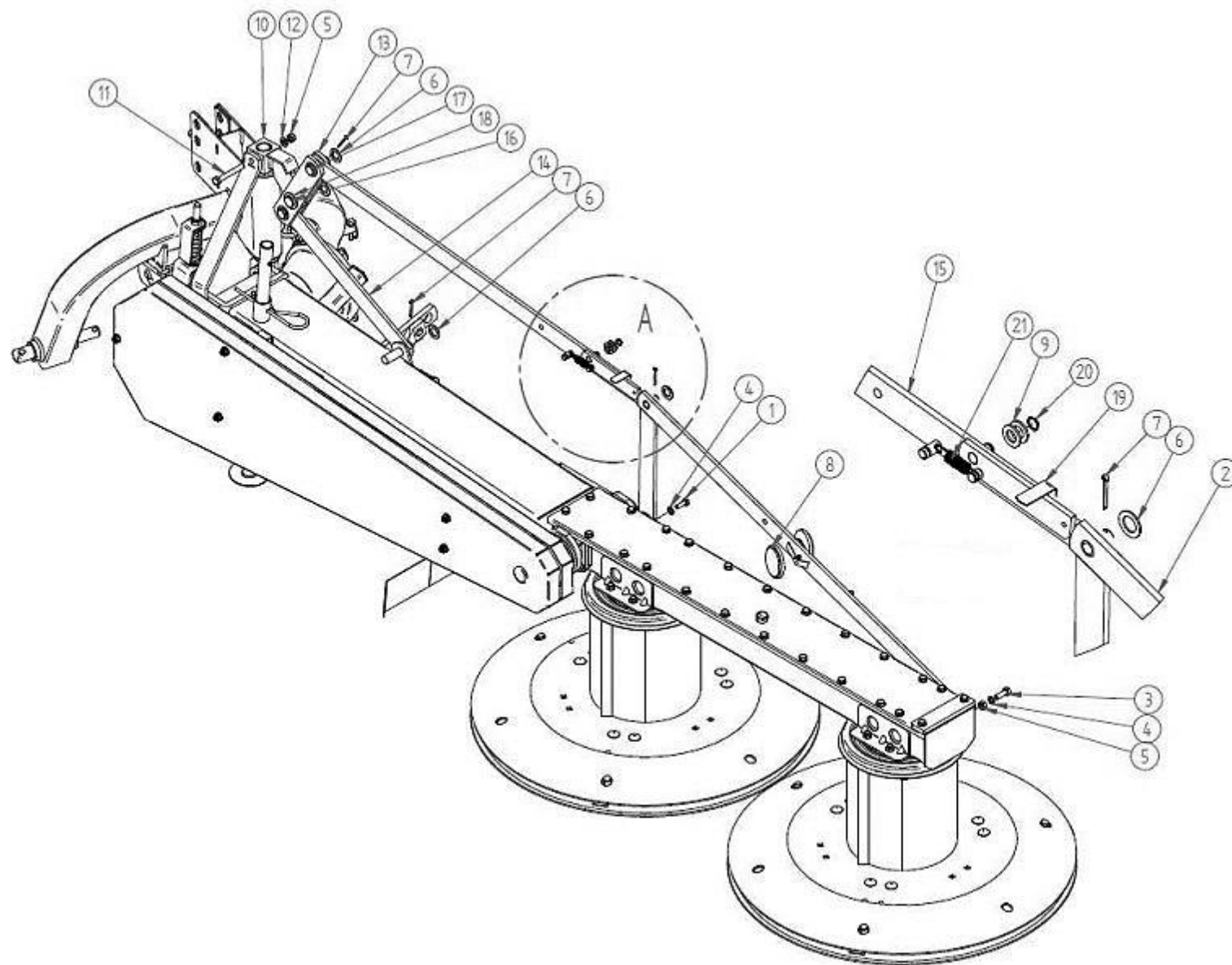
FIGUR 1 – MODEL MED LØFTEANORDNING
