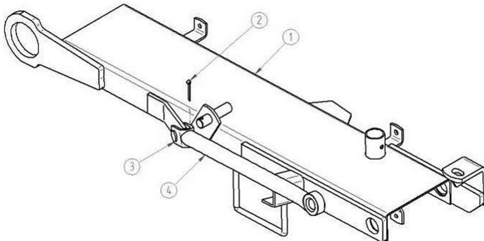
FIGUR 6 – CENTERRAMME, 135
