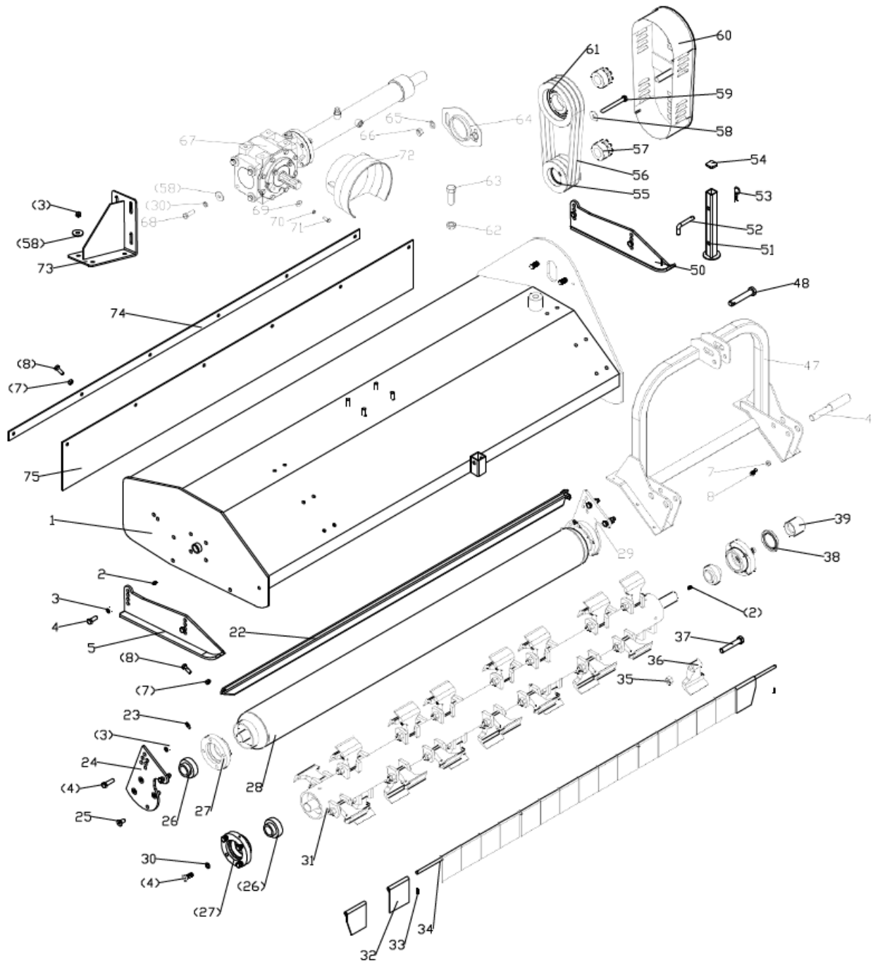
Fig 1 Hovedmaskine
