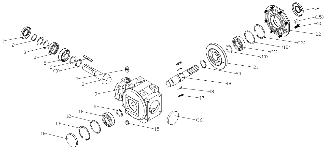
FIG. 3 GEARKASSEDELE
