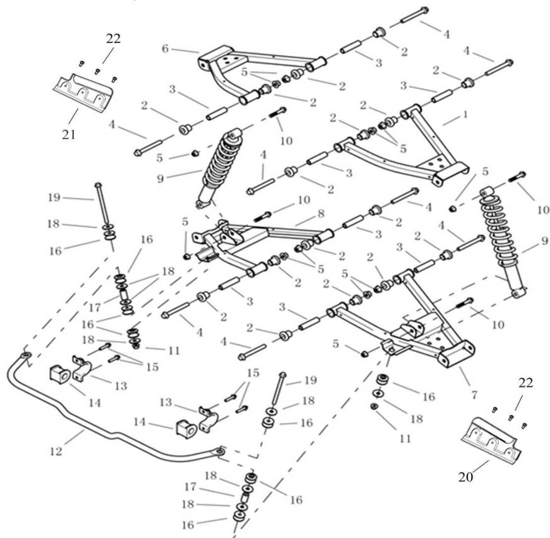
FIGUR 9 – STØDDÆMPE, BAG/ SHOCK ABSORBERS, REAR
