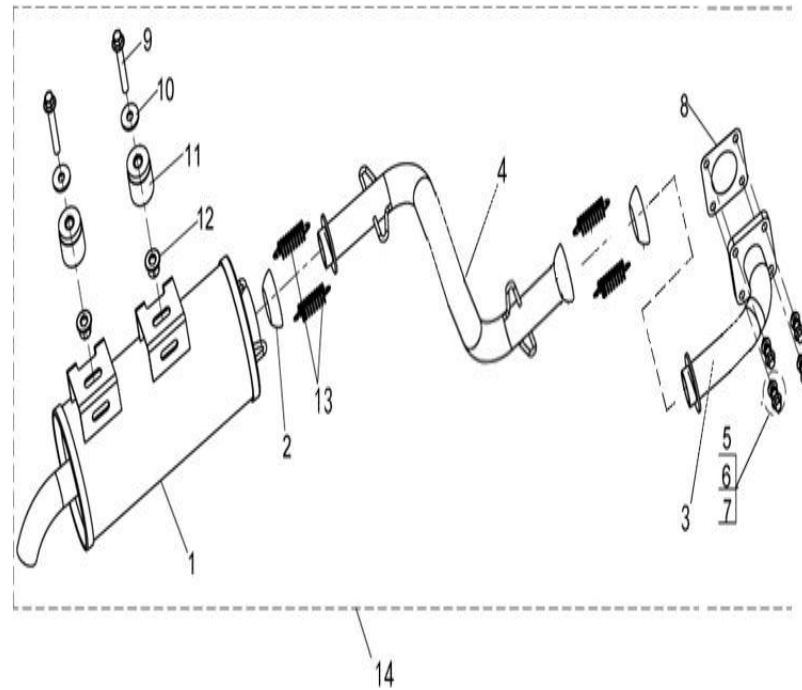
FIGUR E4 – UDSØDNING / EXHAUST
