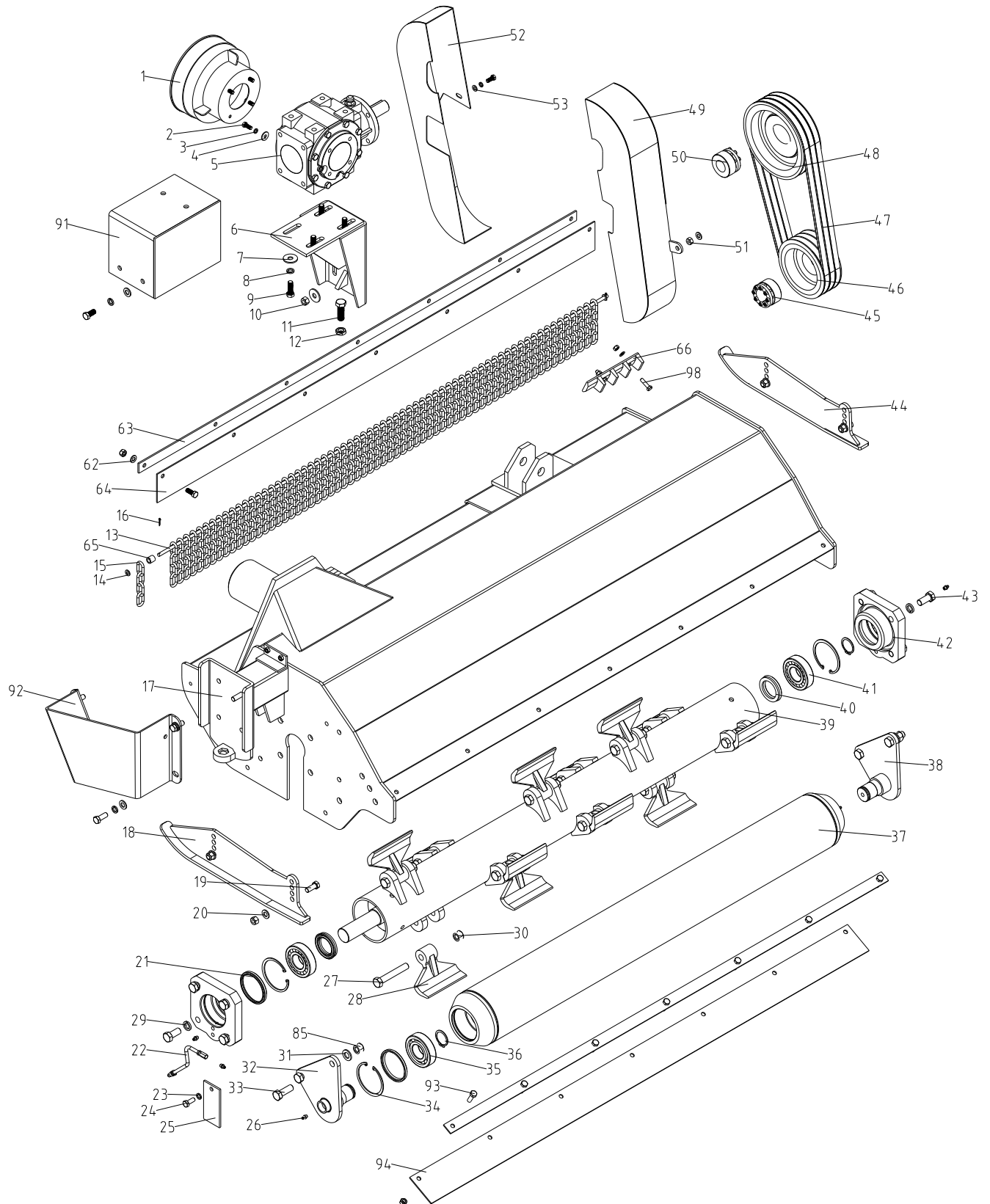
Fig 1 Hovedmaskine
