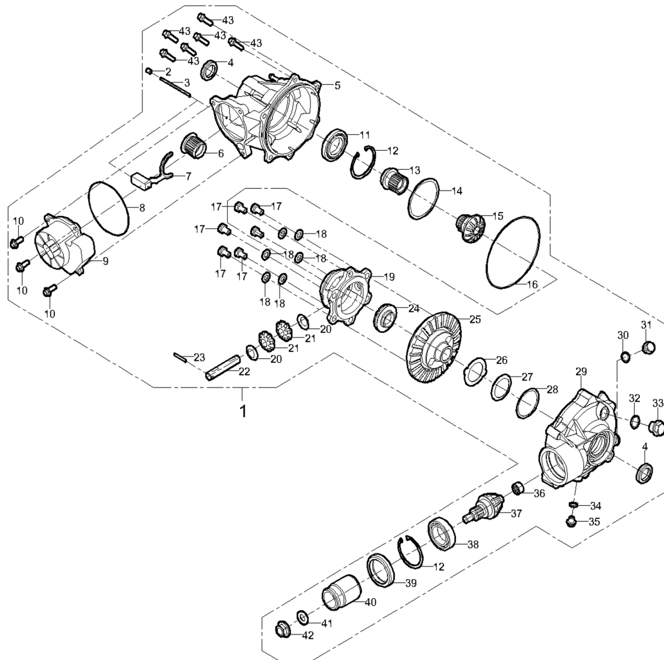
Fig 1.1: Forreste diff/drev-træk/Front drive system assembly
