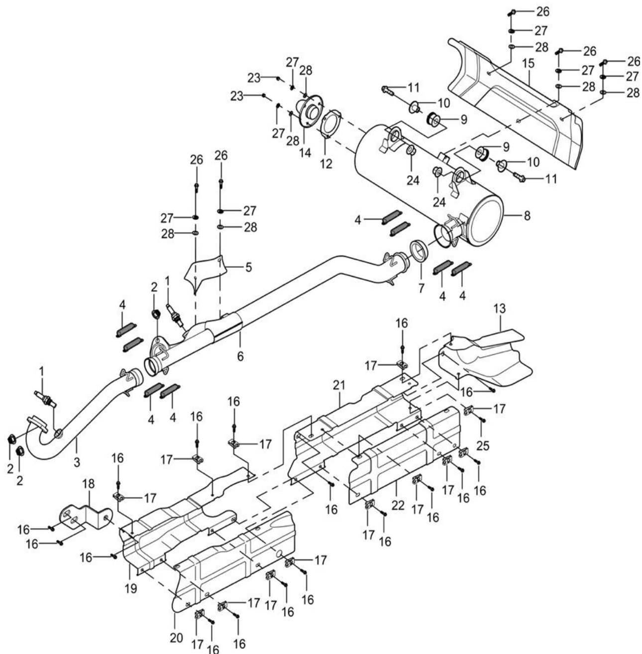
Fig 16: Udstødningssystem "kort"/Exhaust system "short"
