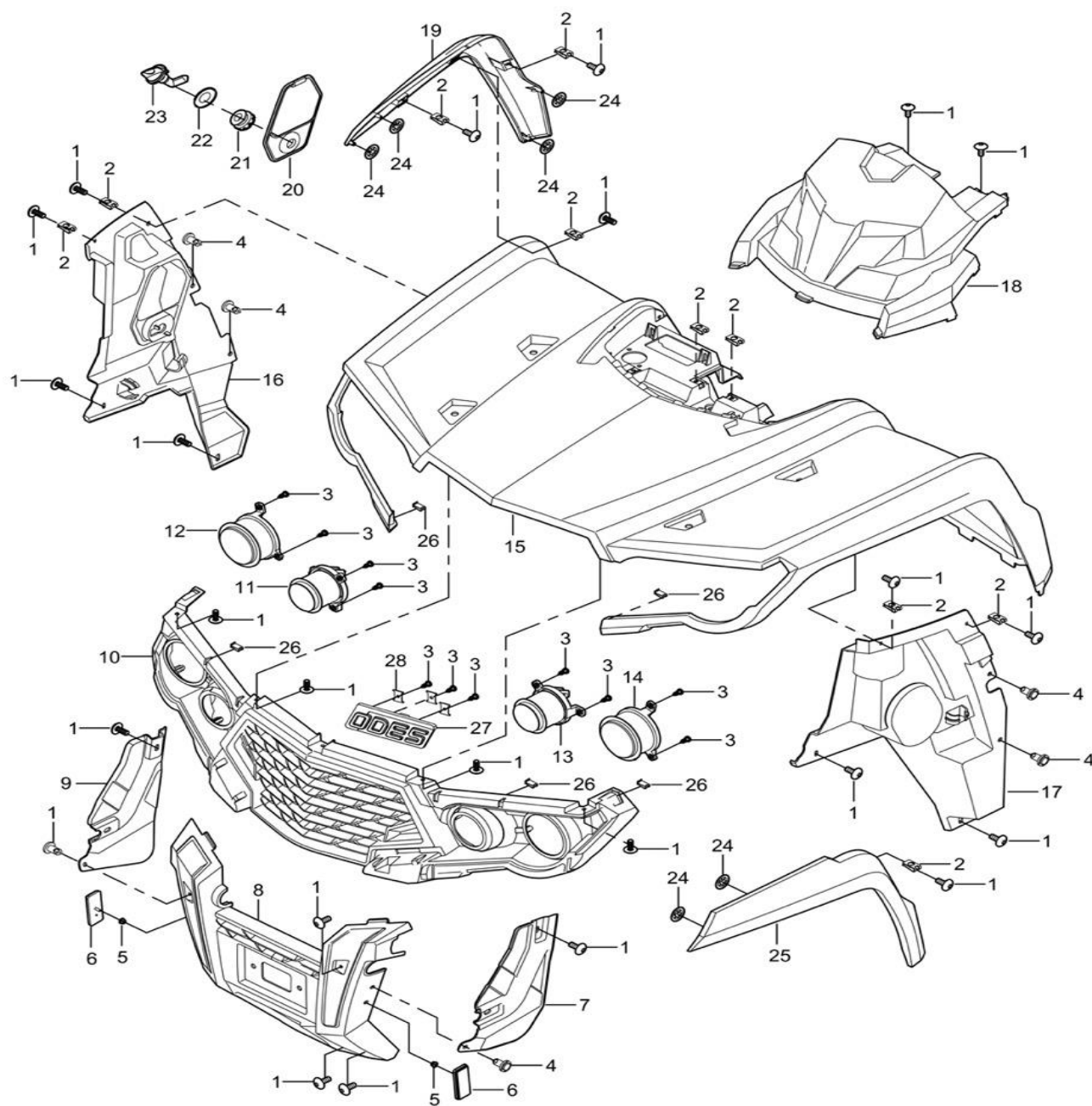
Fig 23: Forskærm, lygter, grill/Headlamp combination
