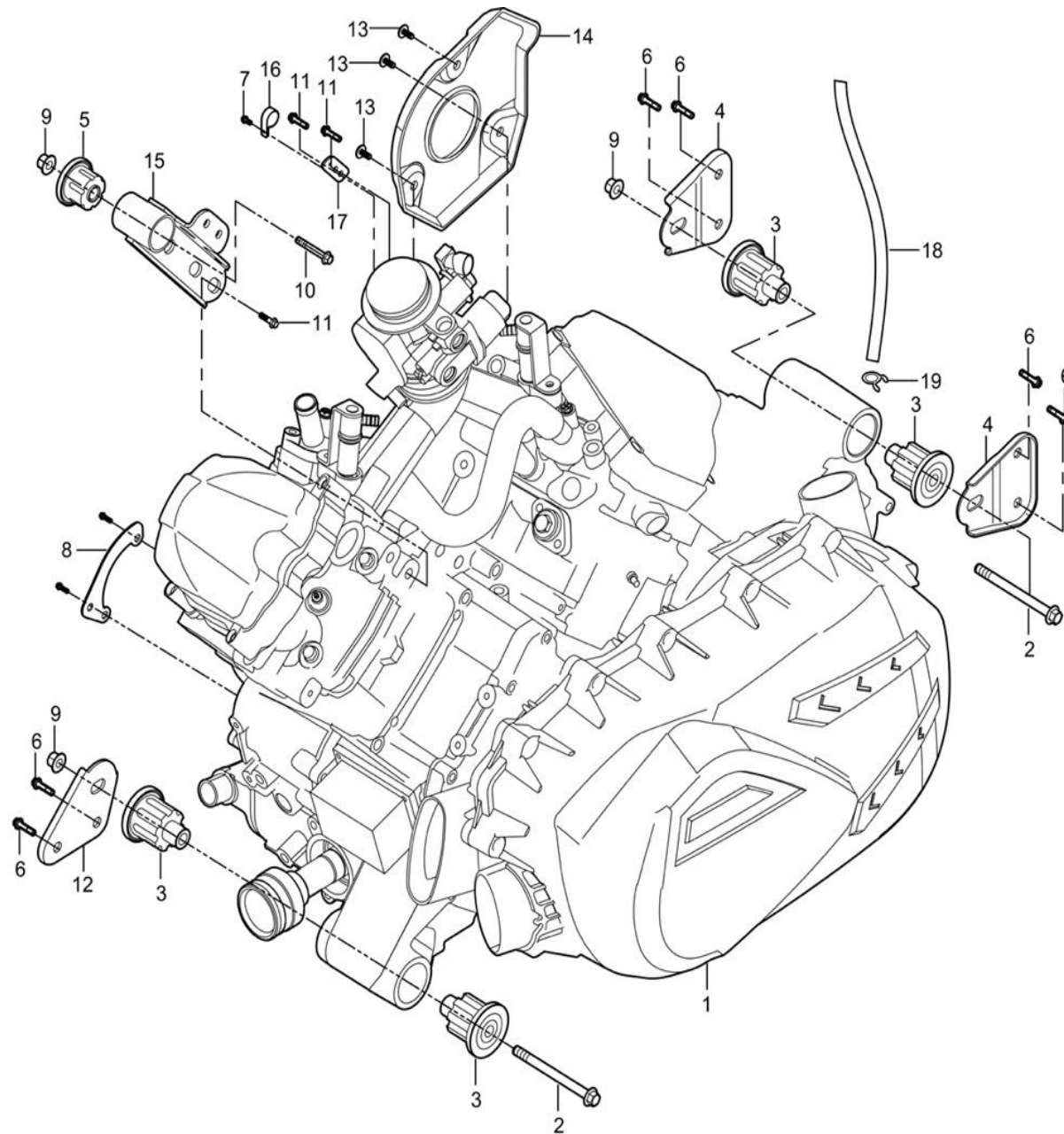
Fig 11: Motor, motorophæng/Engine
