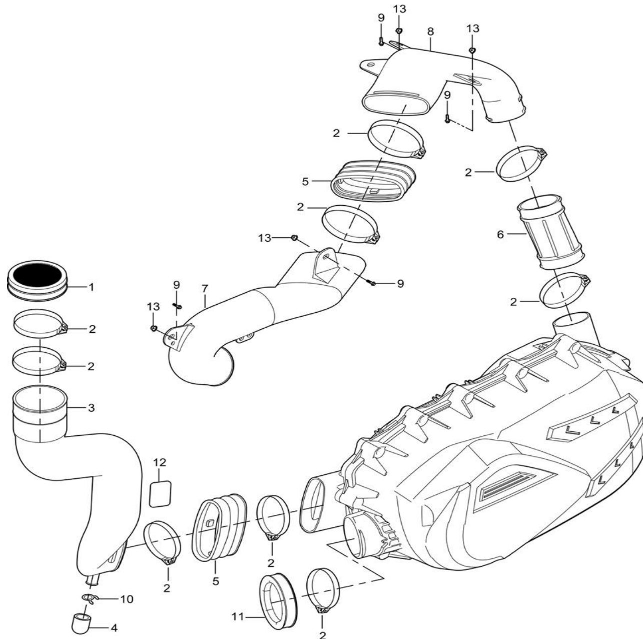
Fig 13: Luftindtag/Air intake CVT
