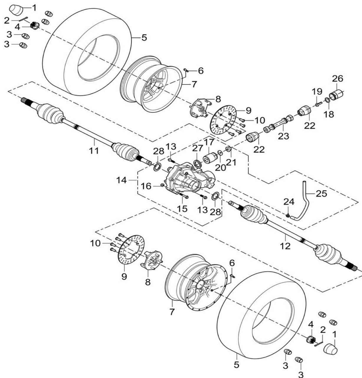
Fig 1: Forreste diff/drev-træk/Front drive system assembly
