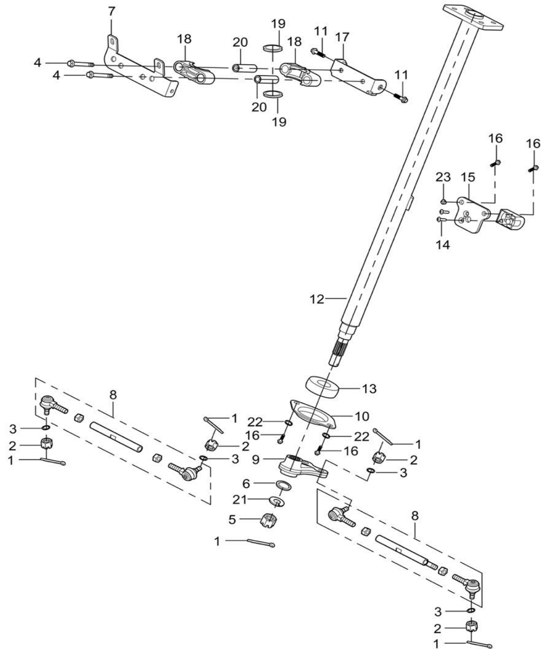
Fig 7: Styretøj uden servo/Steering system without EPS
