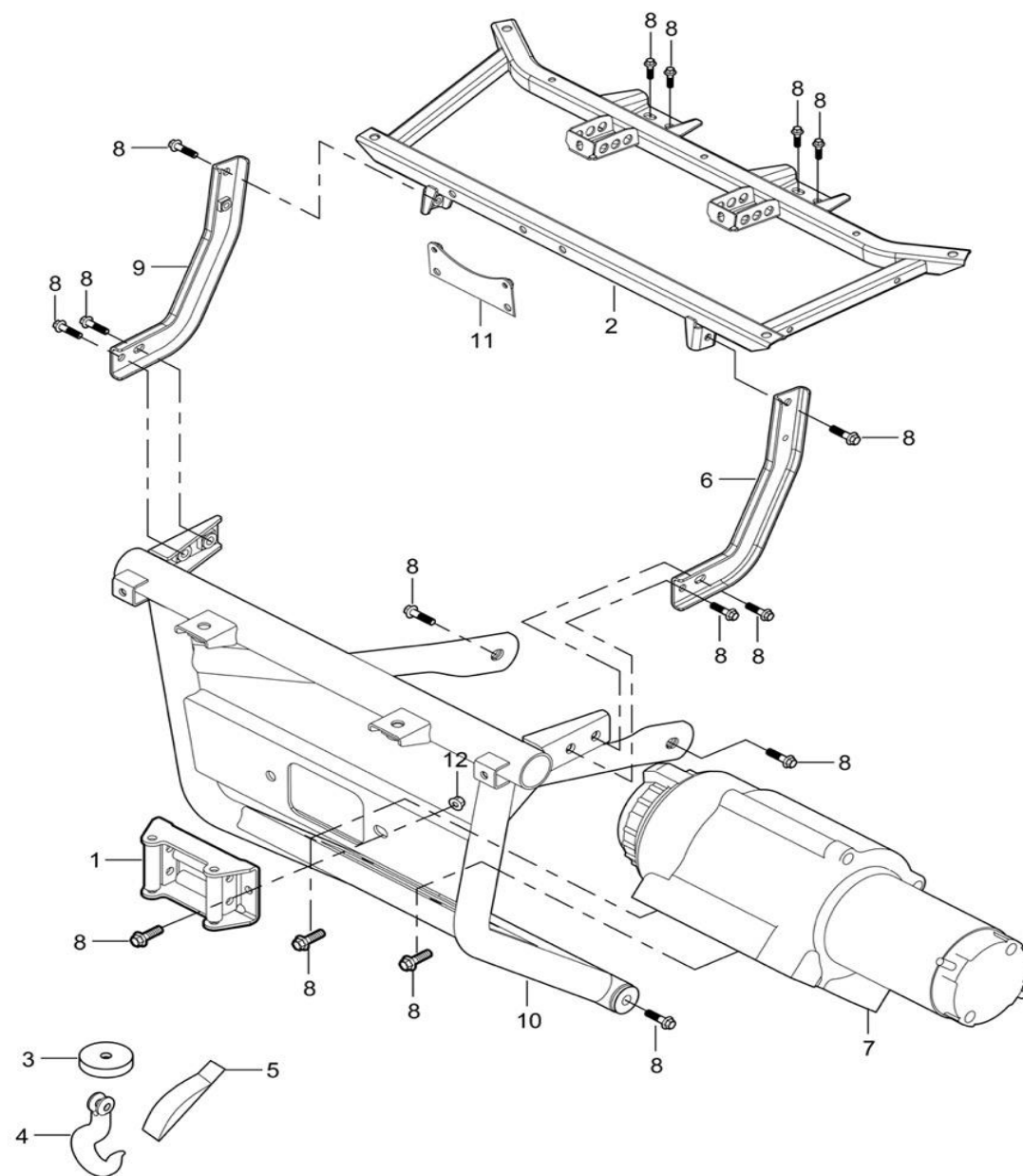
Fig 29: Tilbehør, spil, spilophæng/Optional accessories
