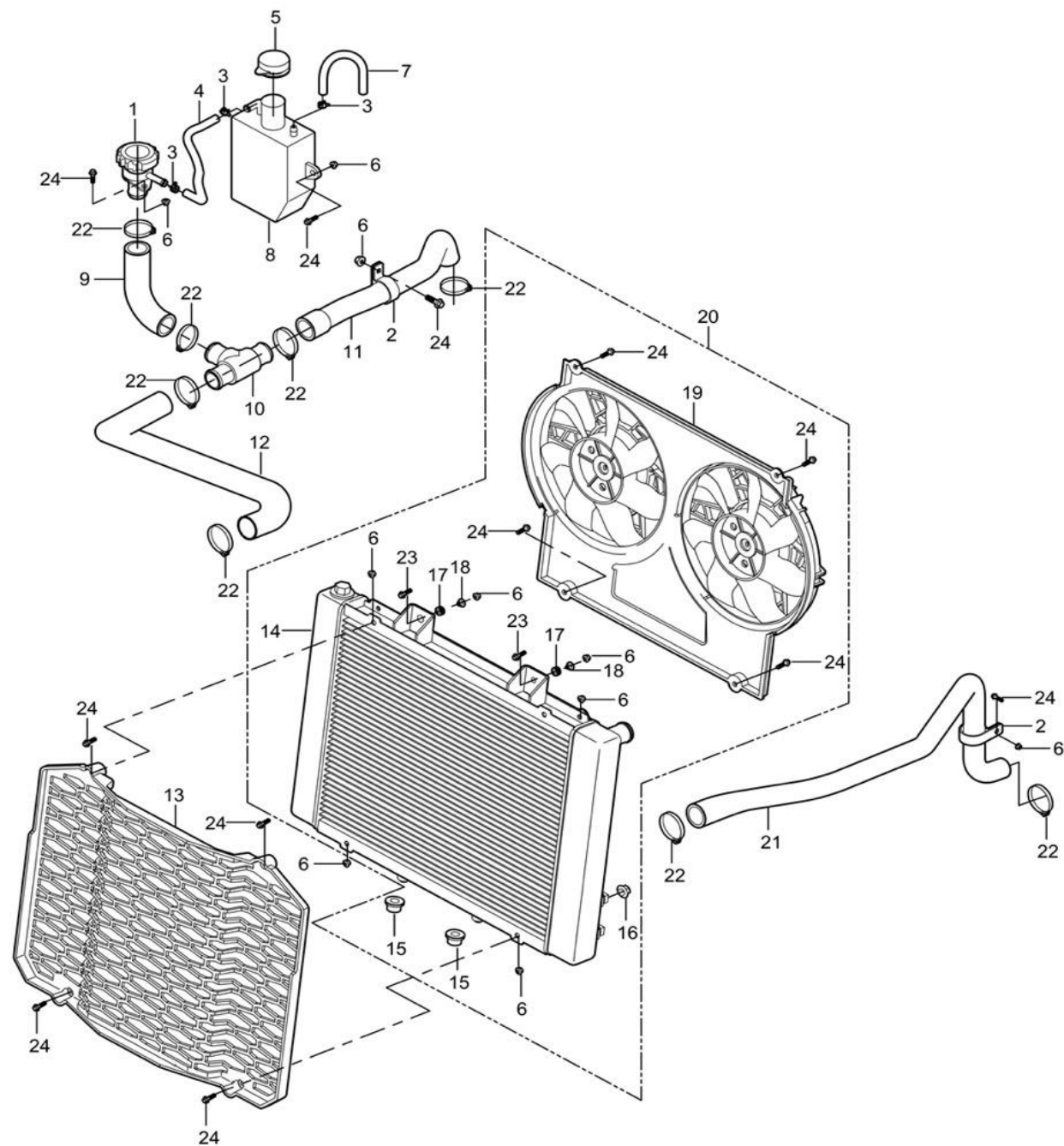
Fig 19: Kølersystem/Cooling system
