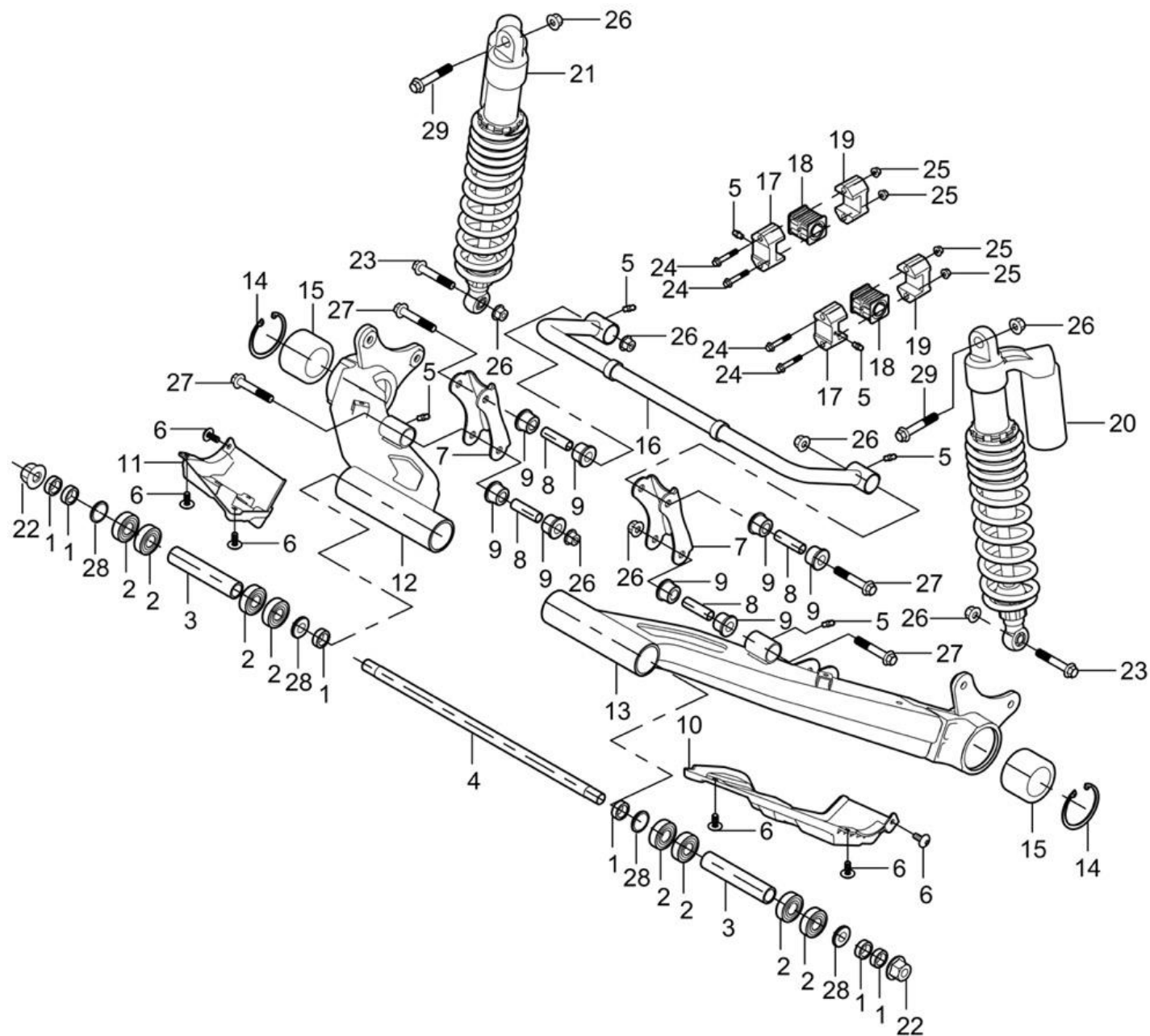
Fig 4: Hjulophæng bagerst/Rear suspension system
