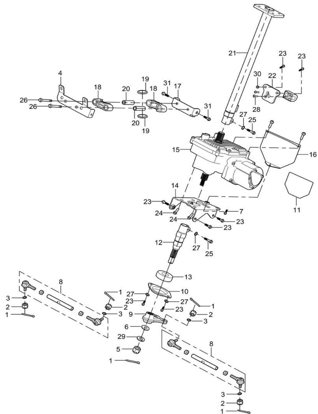
Fig 6: Styretøj med servo/Steering system EPS
