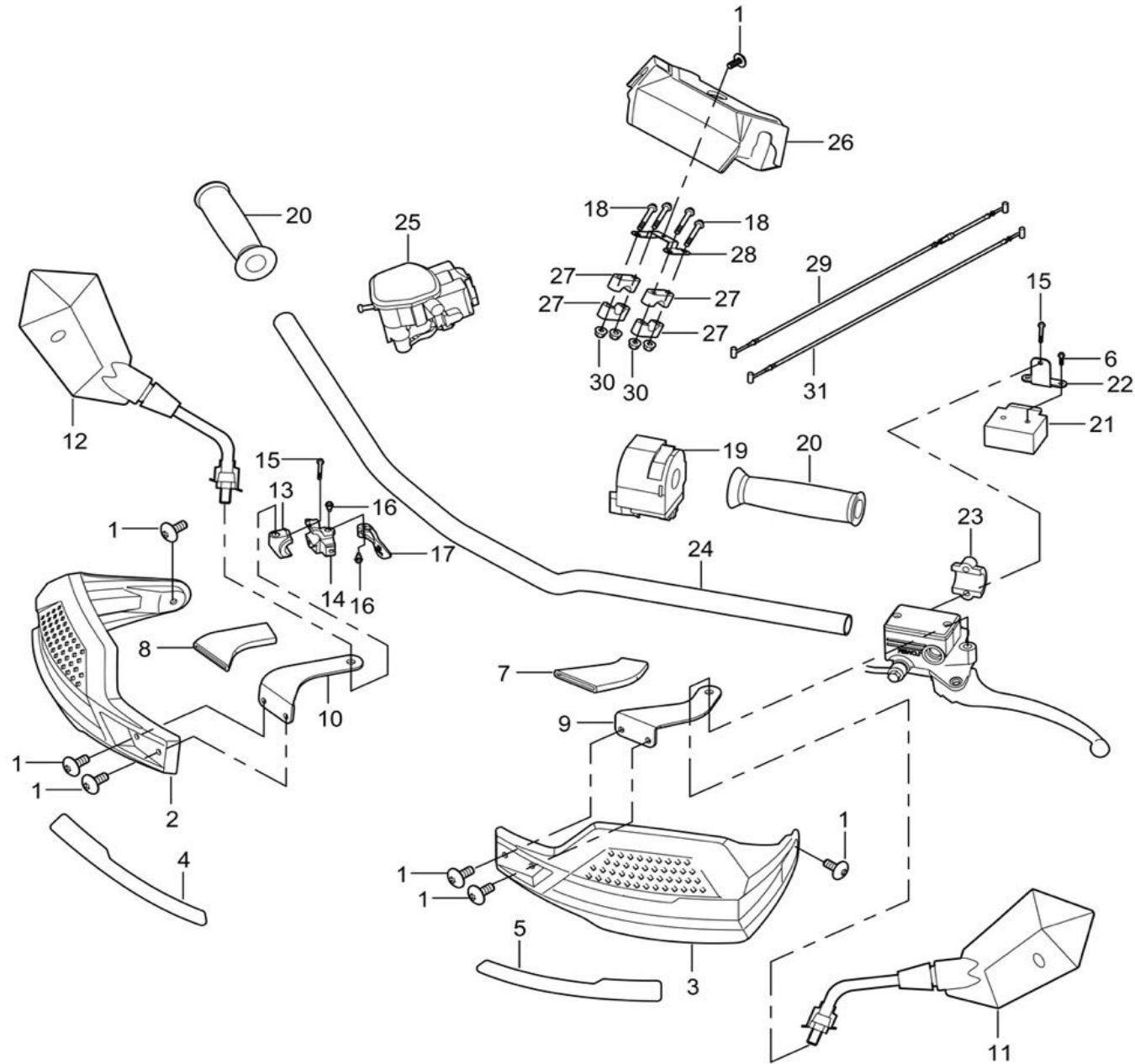
Fig 5: Styr/håndtag/Steering handle
