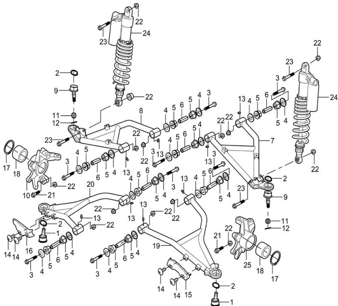
Fig 3: Hjulophæng forrest/Front drive system assembly
