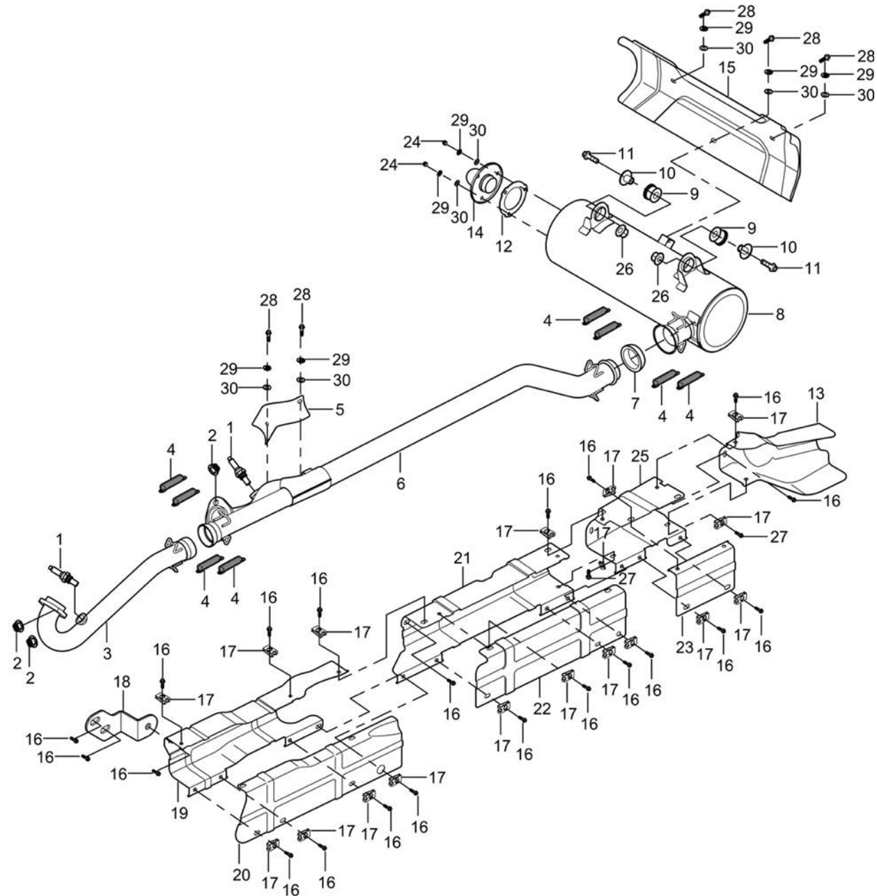
Fig 15: Udstødningssystem "lang"/Exhaust system "long"
