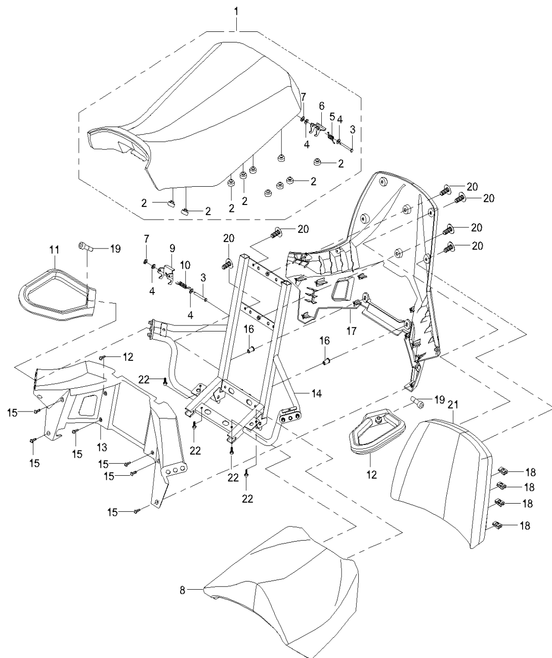
Fig 17: Sæde/beslag "lang model"/Seat "long"
