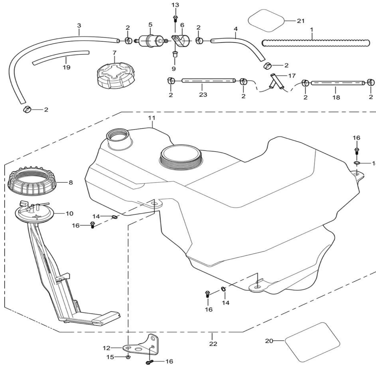
Fig 10: Brændstofsysteem/Fuel system
