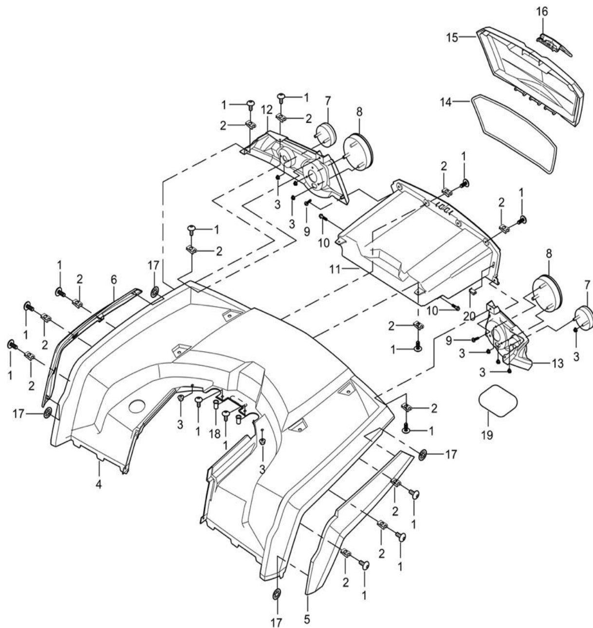
Fig 20: Bagskærm, tilbehør/Rear body assembly
