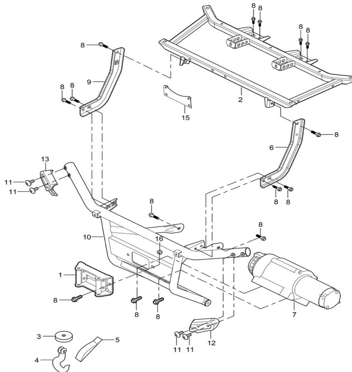
Fig 28: Tilbehør, spil, spilophæng/Optional accessories. T3
