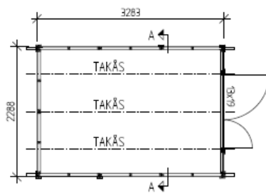
Grundriss
