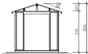
Schnitt
