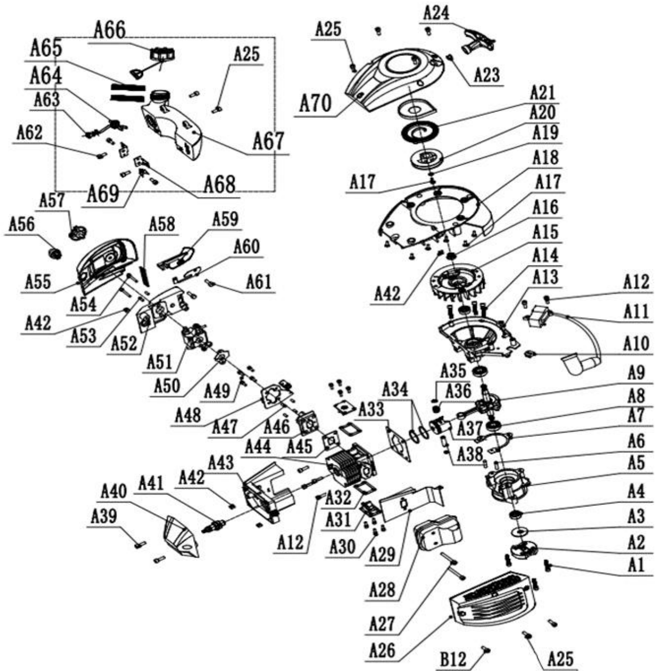
Fig. 1 Motor
