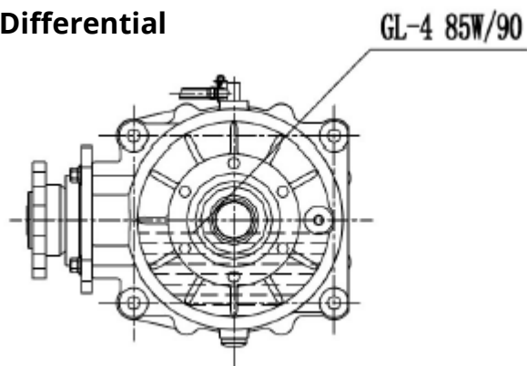
Vorderes Getriebe
