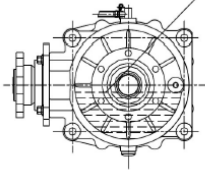
Forreste gearkasse
