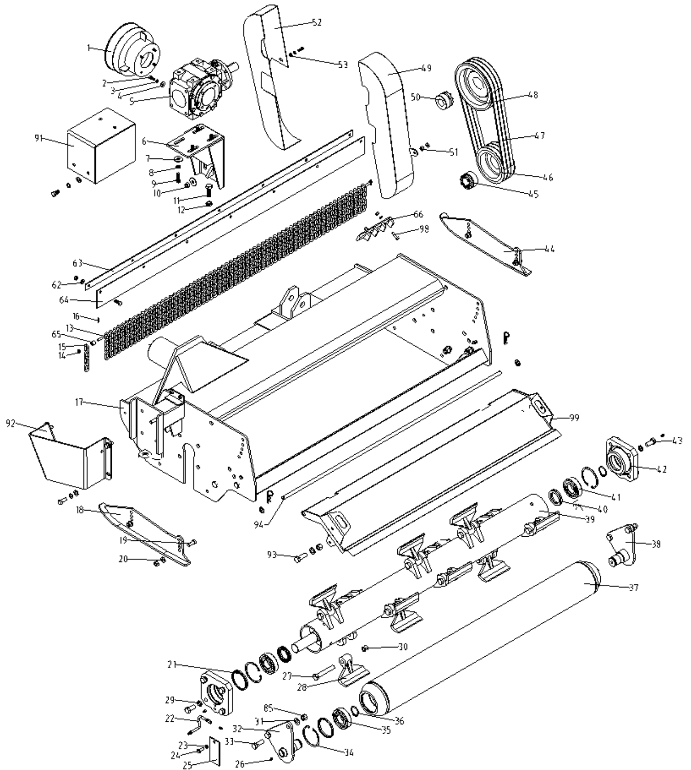
FIG 1, HOVEDMASKINE
