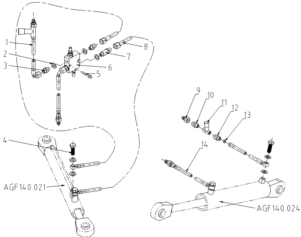
FIG 3, HYDRAULIKSYSTEM
