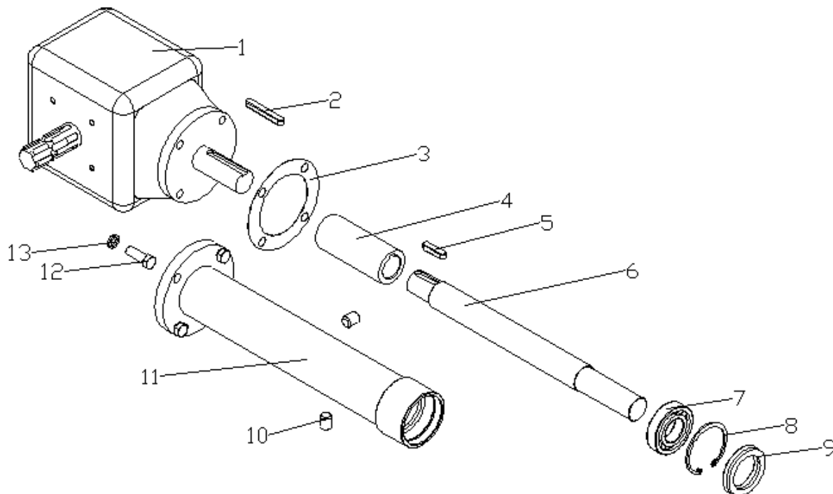
Fig 2. Explosionszeichnung, Getriebe:
