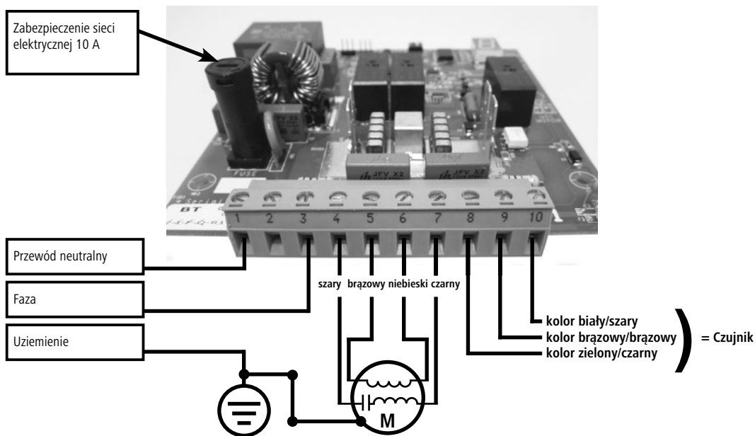
Rysunek 5: Ilustracja podłączenia do HappyCow Swing
