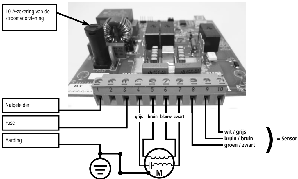
Afbeelding 5: Aansluitschema voor HappyCow Swing
