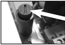
Abbildung 6: Sicherungswechsel für HappyCow Swing
