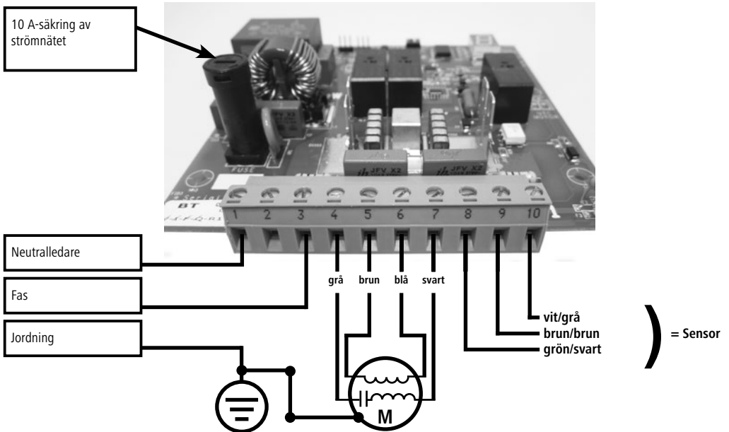
Bild 5: Anslutningsbild för HappyCow Swing
