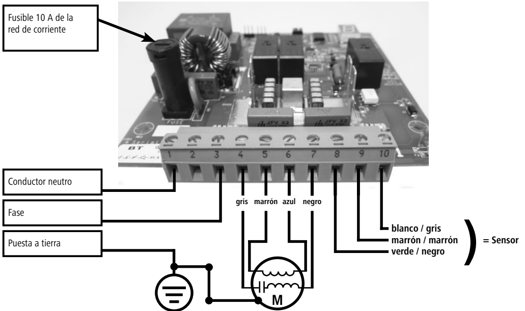
Figura 5: Esquema de conexiones para HappyCow Swing
