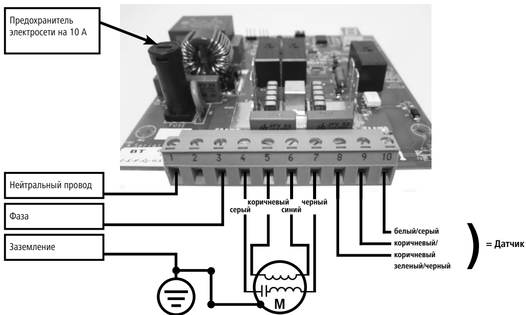
Рисунок 5: Схема электрических подключений для моделей HappyCow Swing
