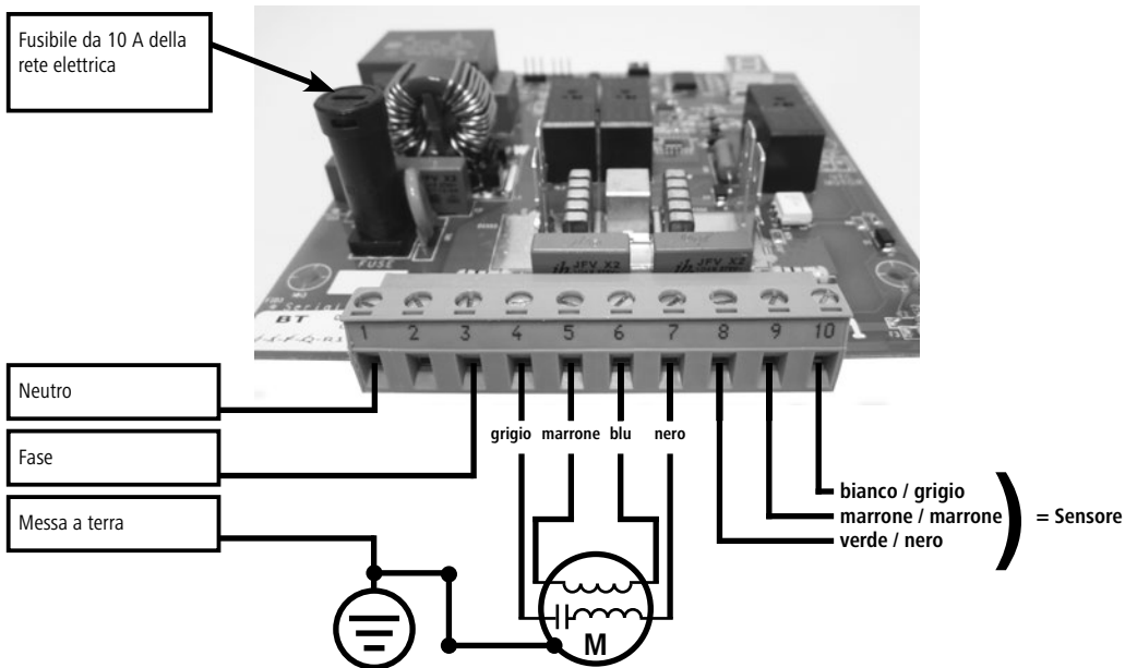
Figura 5: Schema dei collegamenti per HappyCow Swing
