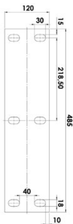
Рисунок 2: Схема расположения отверстий
