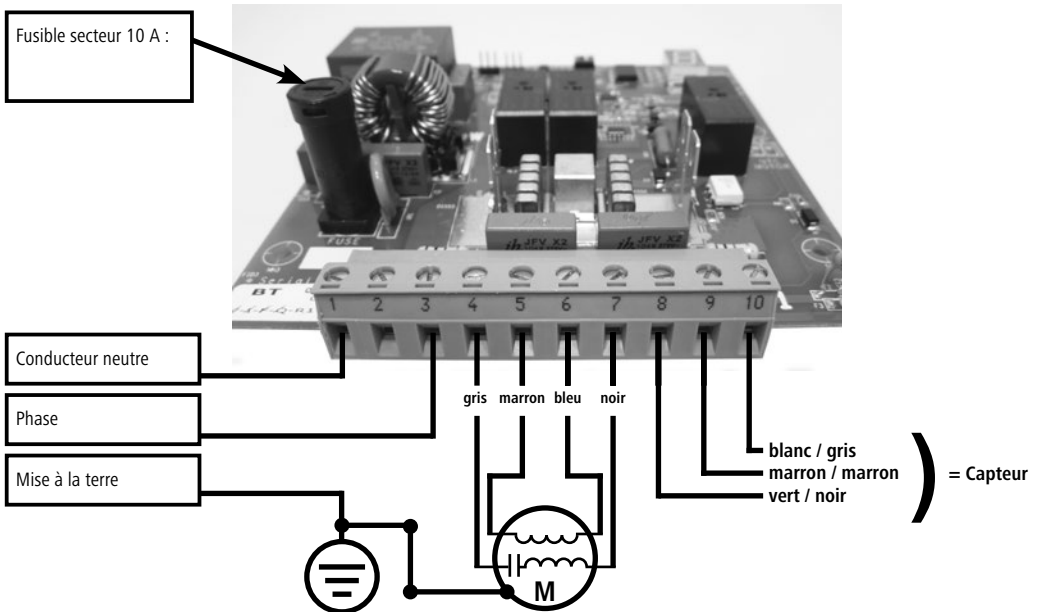
Figure 5 : schéma de raccordement pour HappyCow Swing
