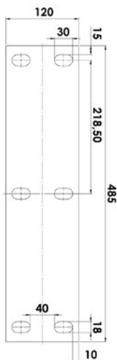
Afbeelding 2: Boorsjabloon
