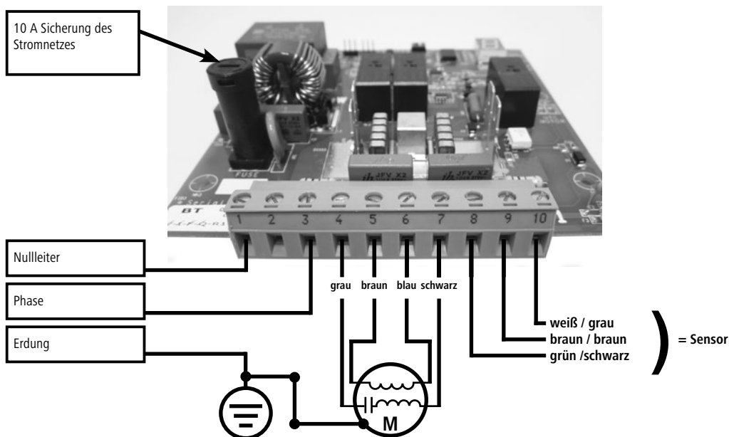
Abbildung 5: Anschlussbild für HappyCow Swing
