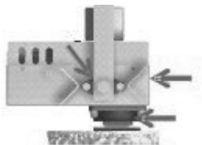
Bild 7 - smörjpunkter på borstlagret © Agricow srl
