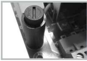
Rysunek 6: Wymiana bezpiecznika w urządzeniu HappyCow Swing
