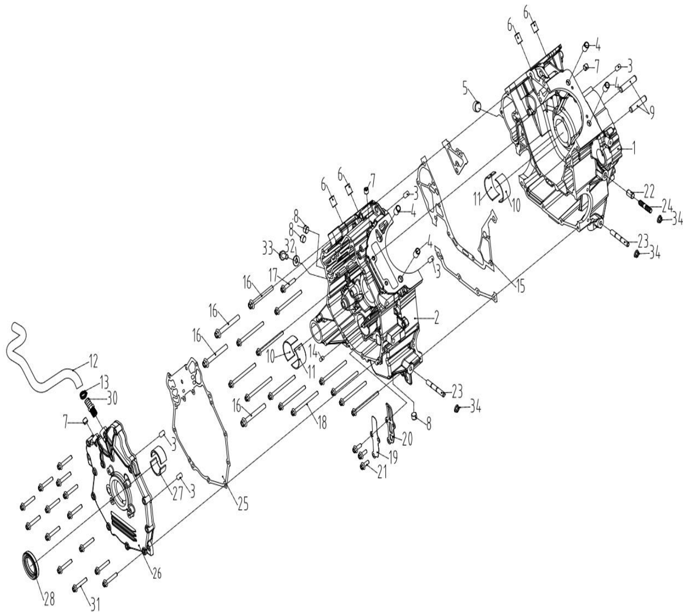
Fig 3: Krumtaphus, lejer / Crankcase
