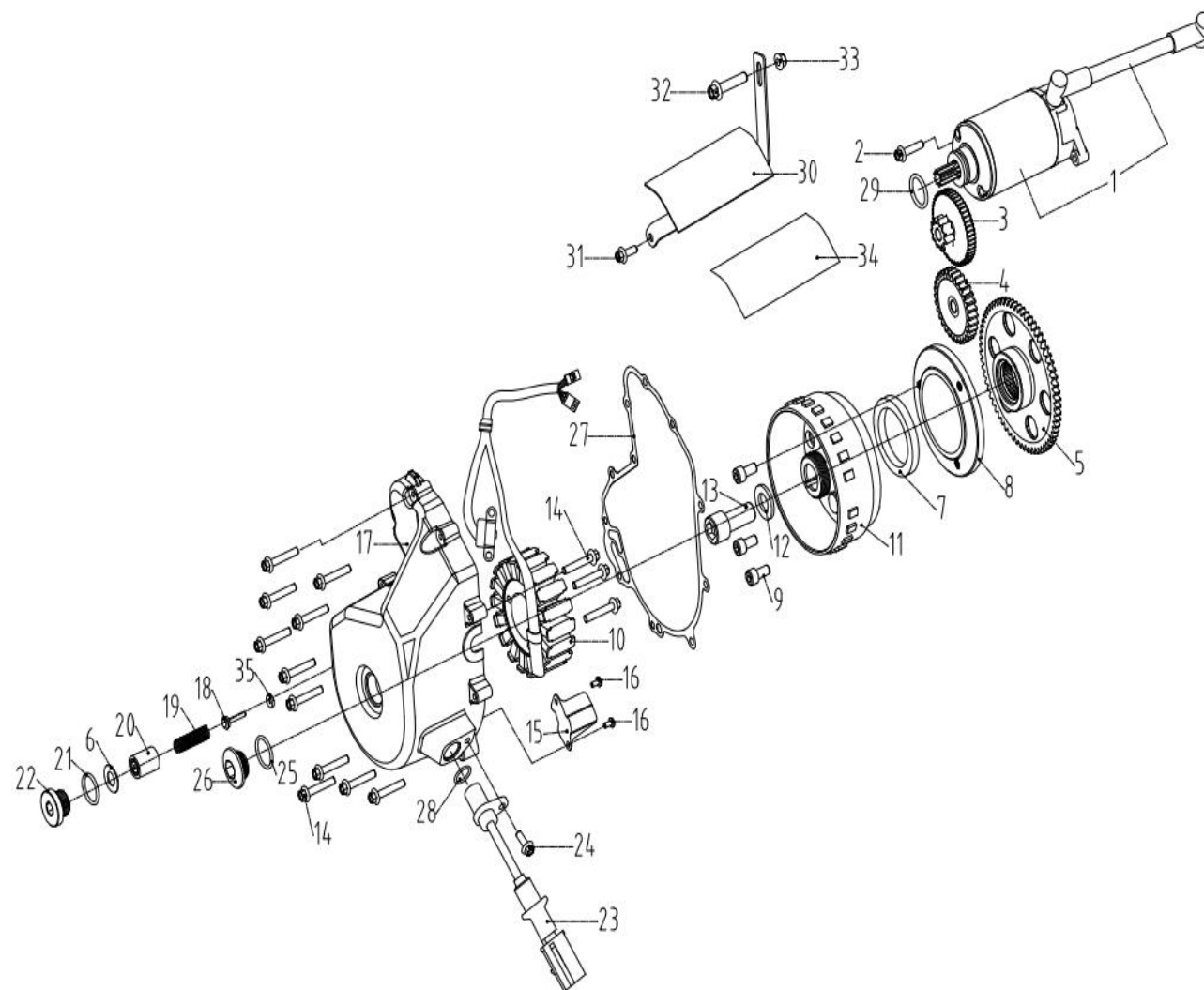
Fig 5: Starter, starterdrev og generator / Magneto
