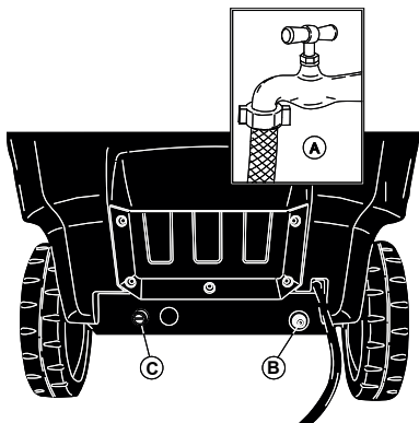
Подключение воды.
