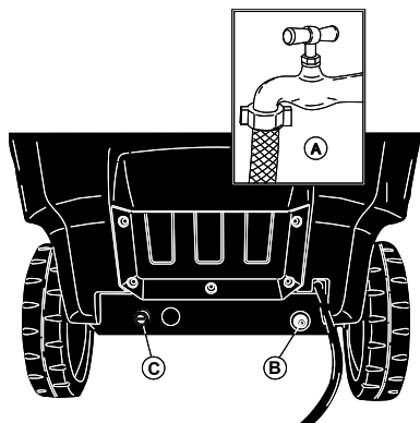
Conexión hídrica.
