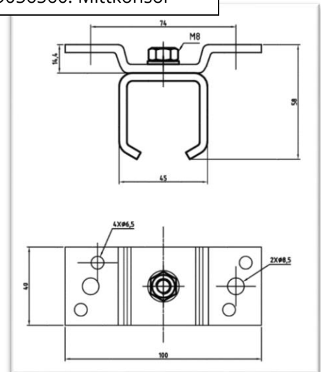
9056560: Mittkonsol
