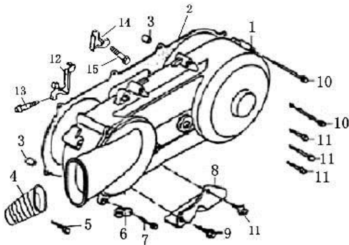
FIG.7 Sidedæksel
