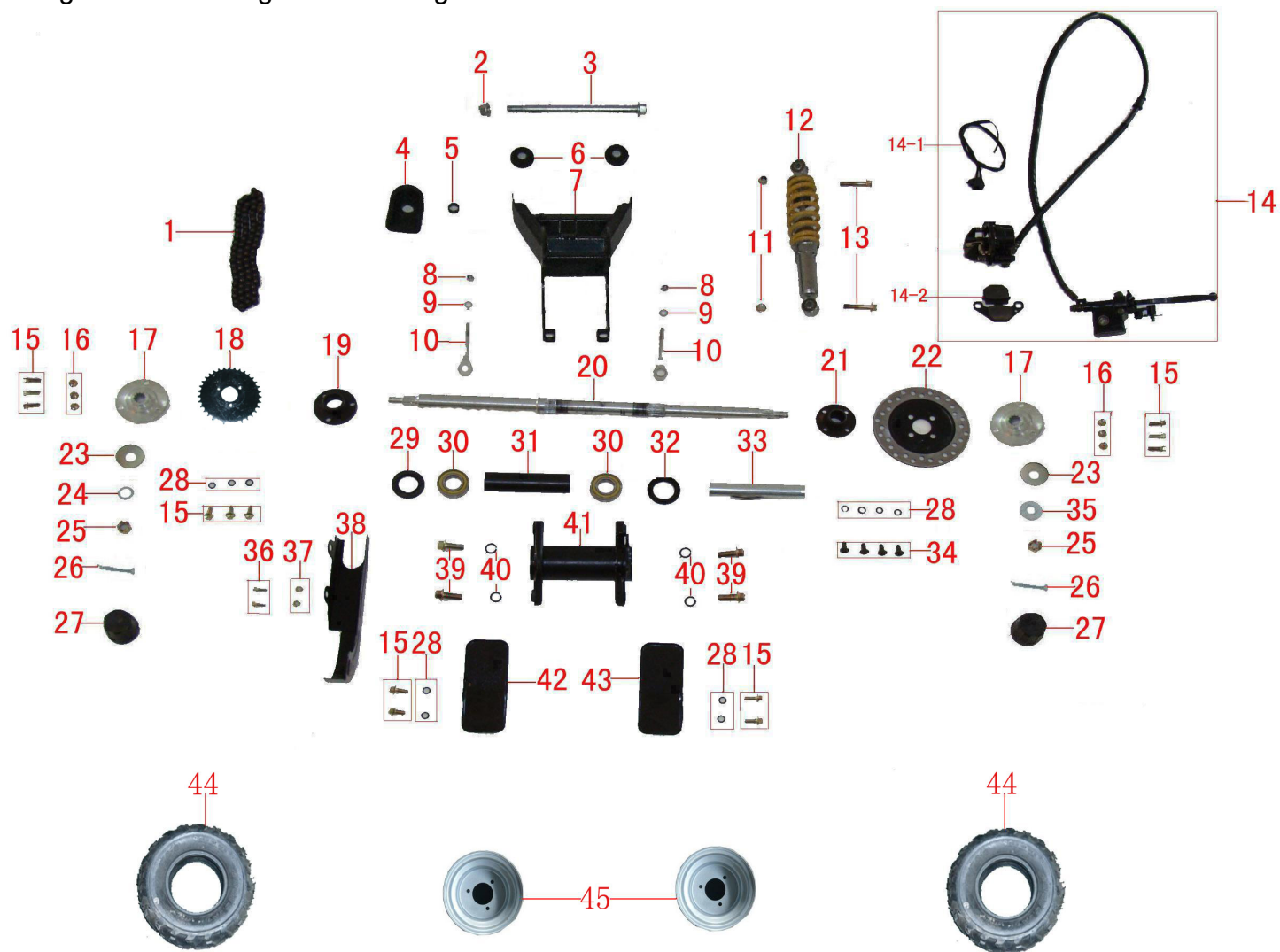
Fig 3: bagerste svingarm / rear swingarm / Schwingarm hinten
