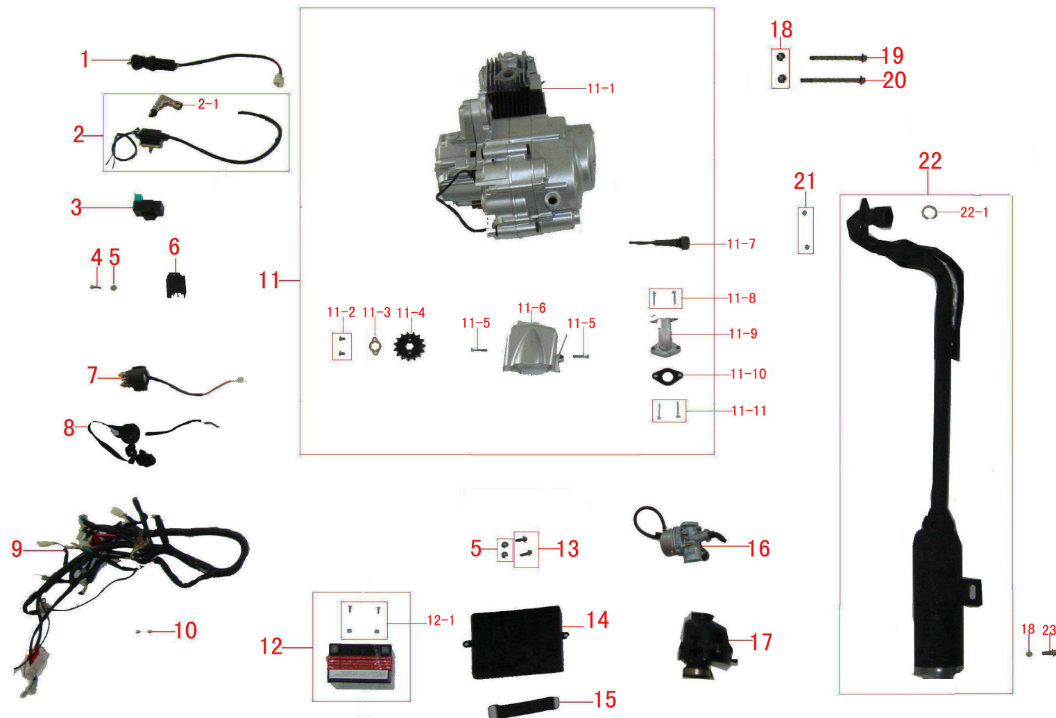
Fig 5: Elektriske dele & motor komponenter / electricals & engine parts / Elektrische Teile & Motorkomponenten
