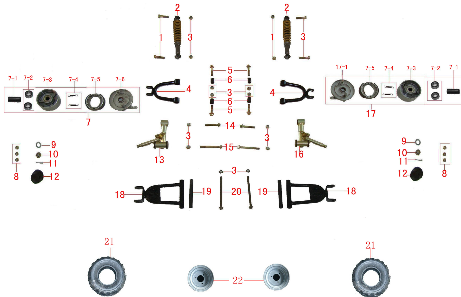
Fig 4: Forhjulsophæng / front suspension / Vorderradaufhängung
