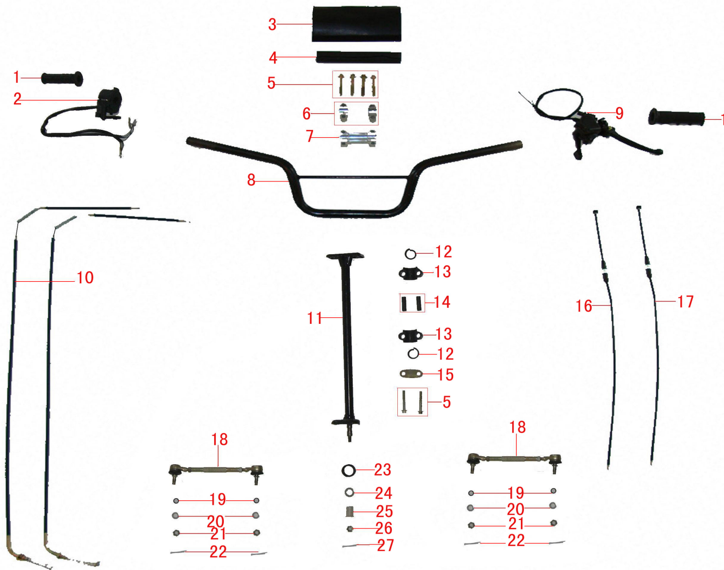
Fig 6: Styringssystem / steering system / Steuerungssystem
