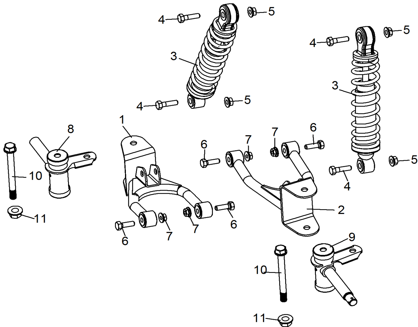
FIG.21 Forhjulsophæng
