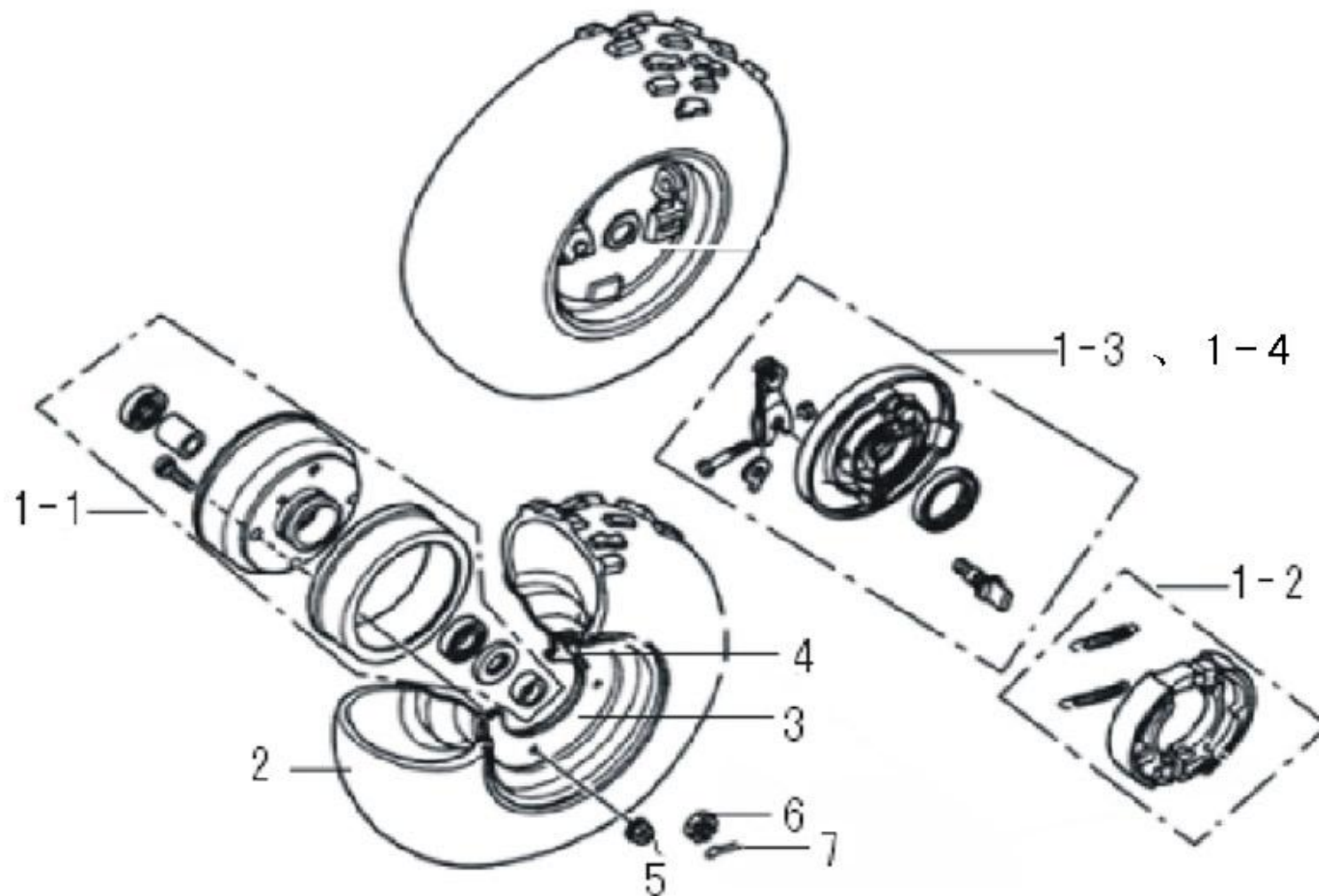
FIG.18 Forhjul & nav
