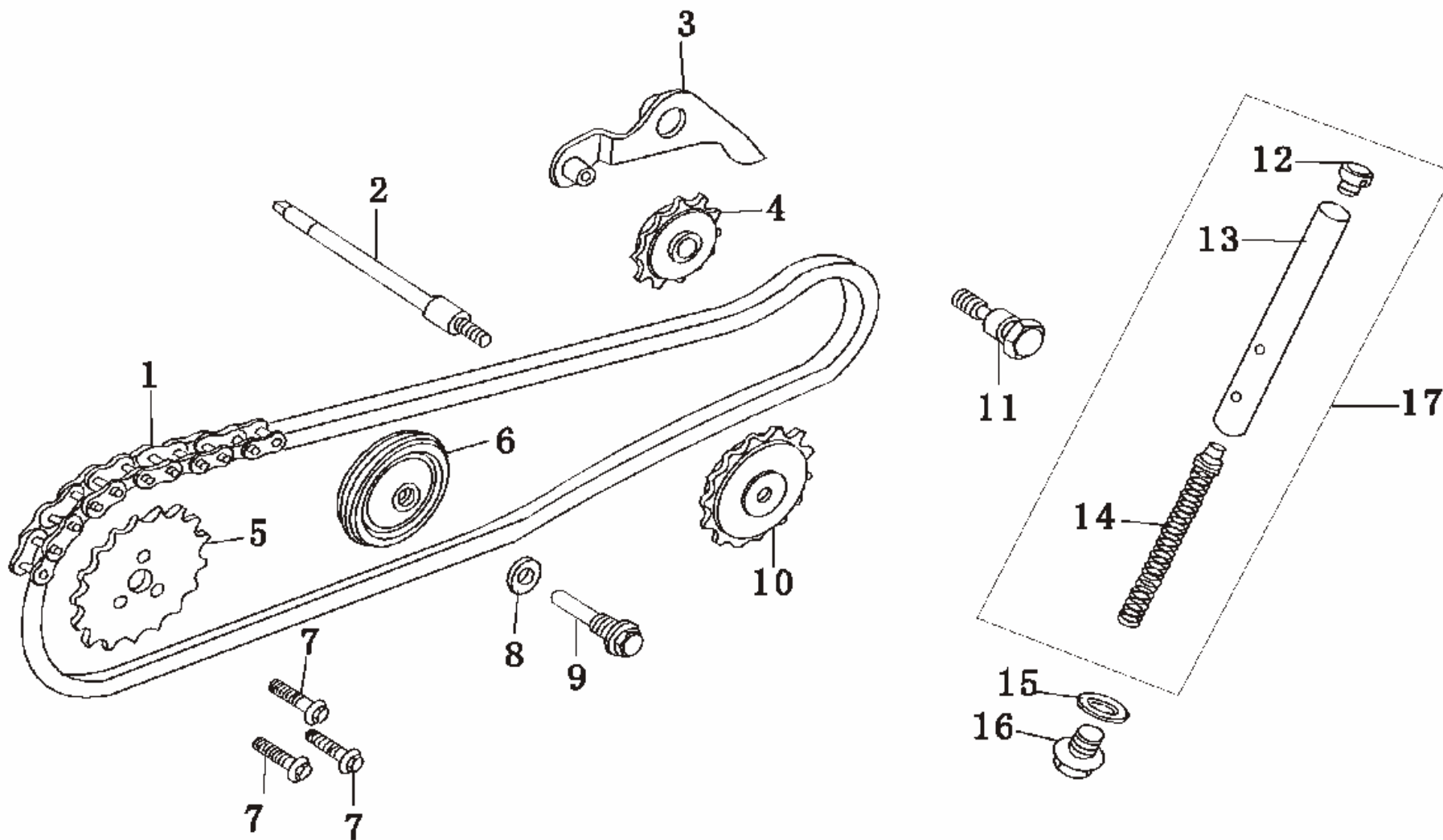
FIG.4 Knastkæde
