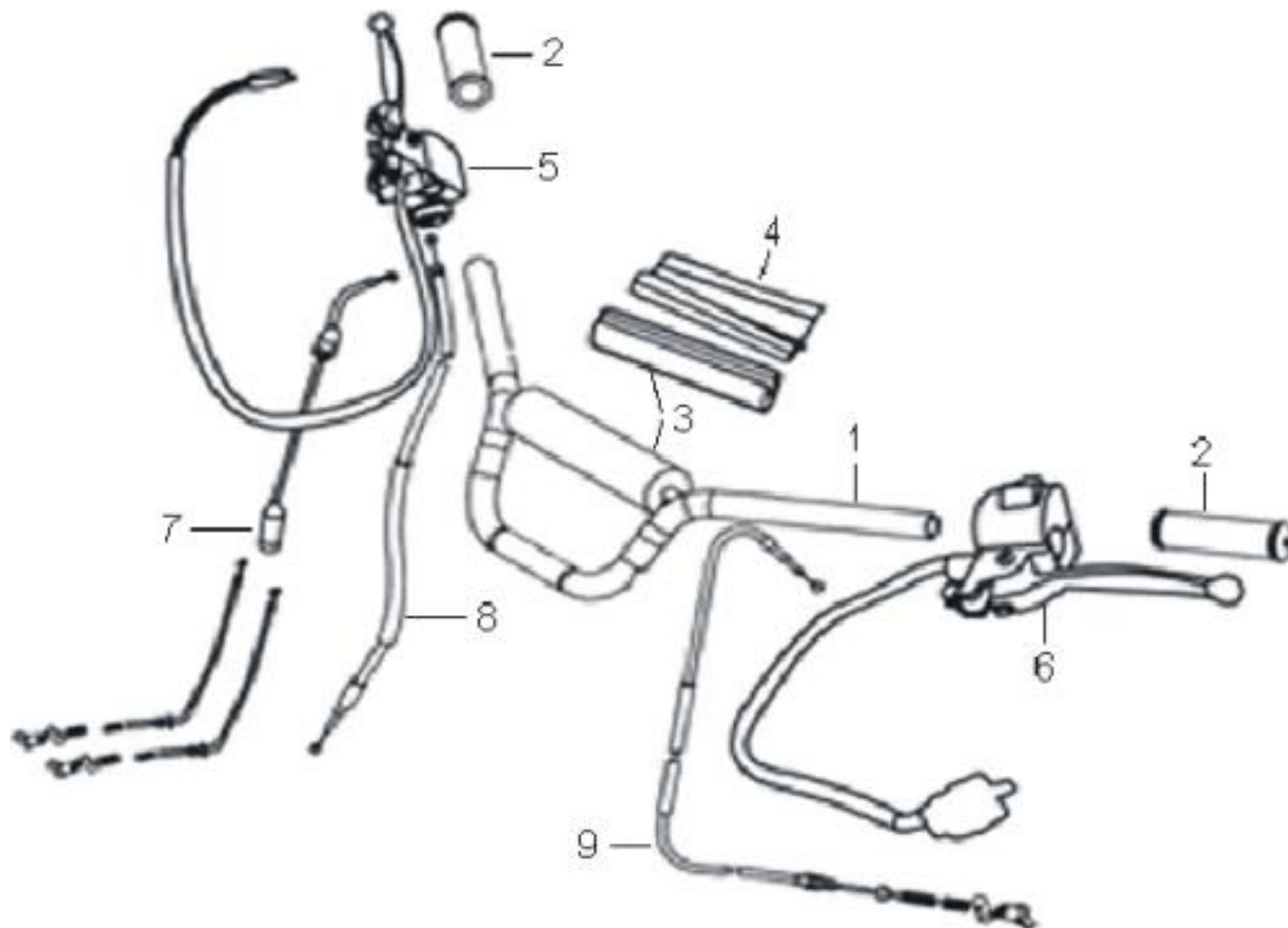
FIG.20 Styr & greb
