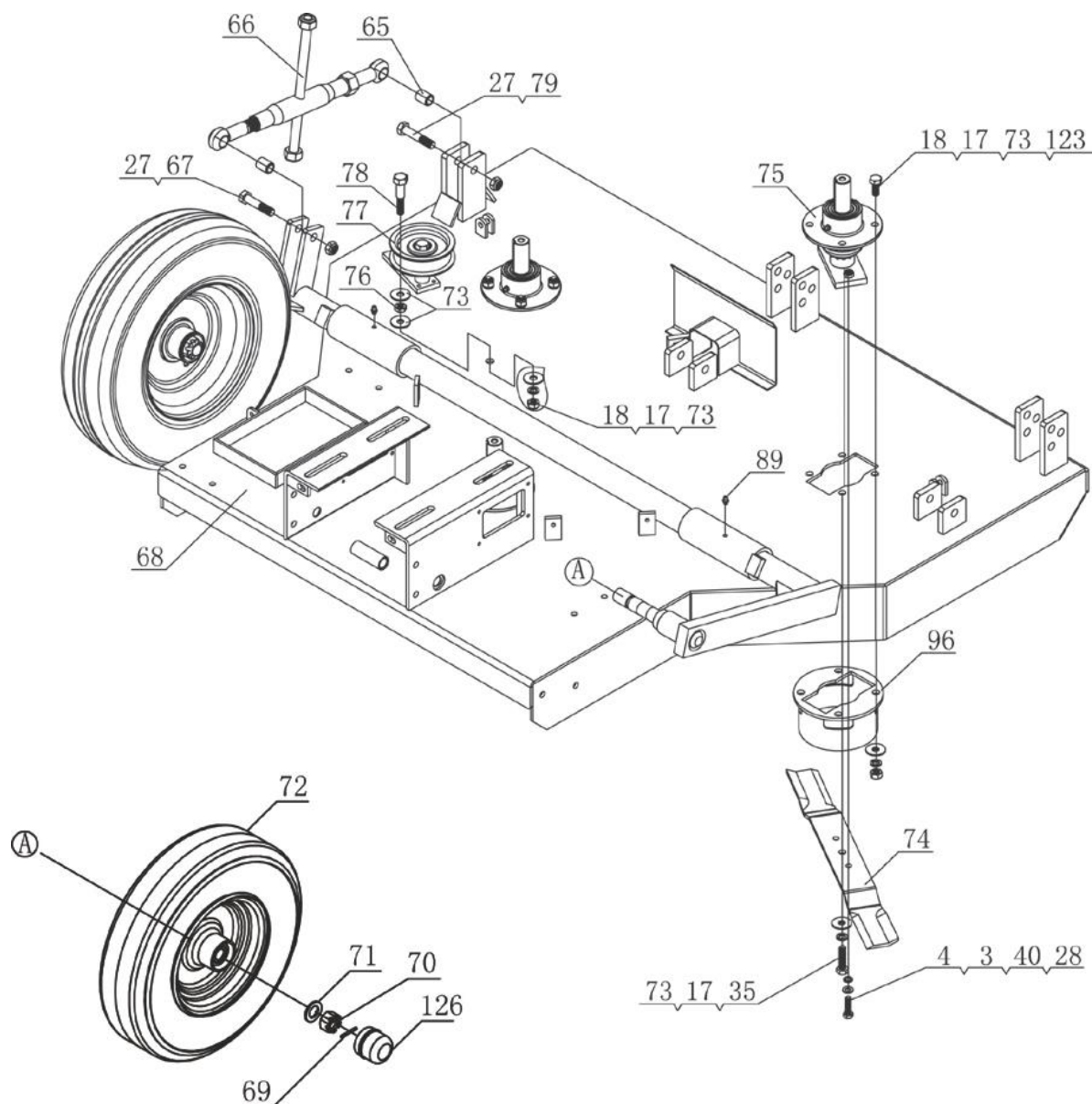
FIGUR 2 - KLIPPBORD
