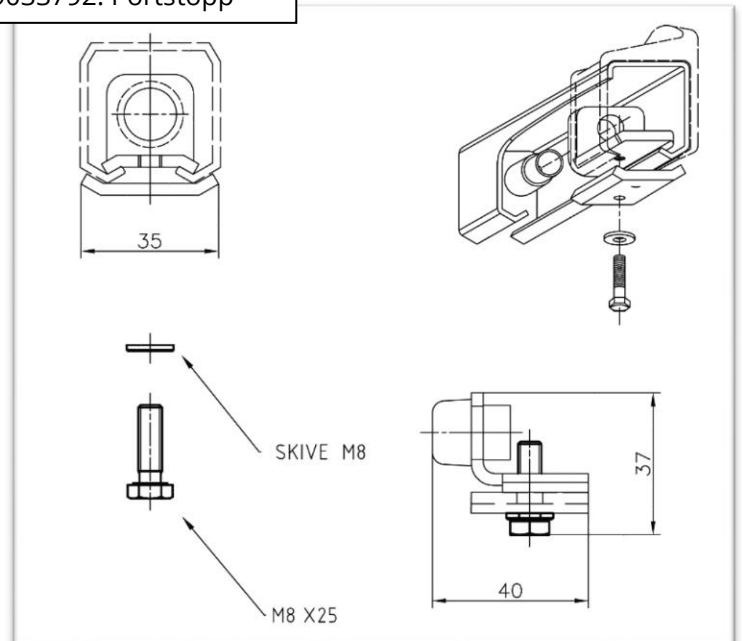
9033792: Portstopp
