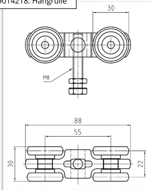
9014218: Hängrulle
