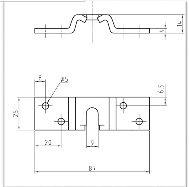
9033791: Bärplatta
