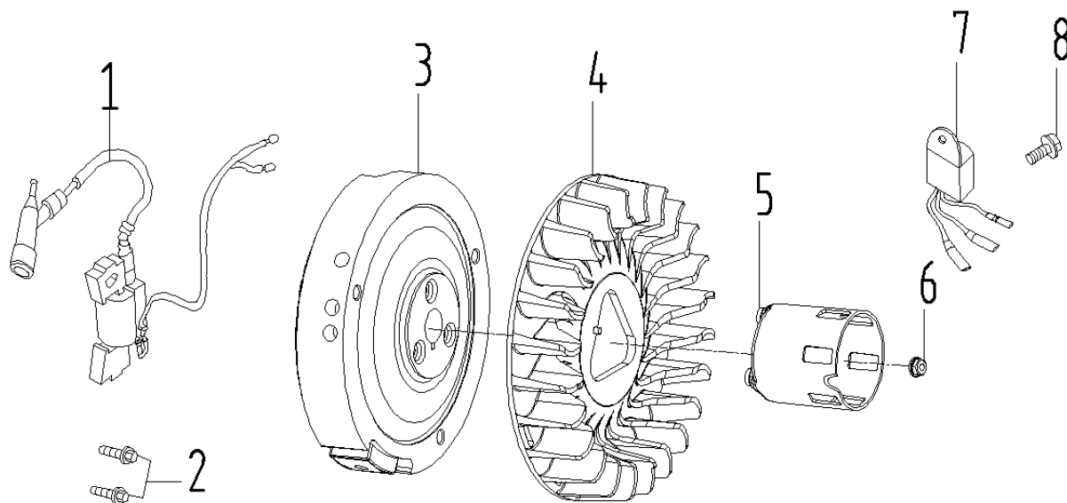
MOTOR FIGUR 9 – SVINGHJUL / FLYWHEEL
