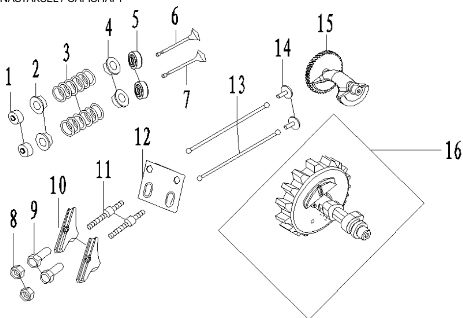
MOTOR FIGUR 5 – KNASTAKSEL / CAMSHAFT
